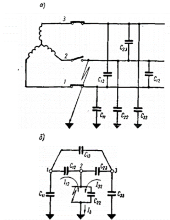
Рисунок 5.4 – Схема сети с по фазным АГТВ C_e ) и схема протекания емкостных токов при обрыве дуга в выключателе (б)
