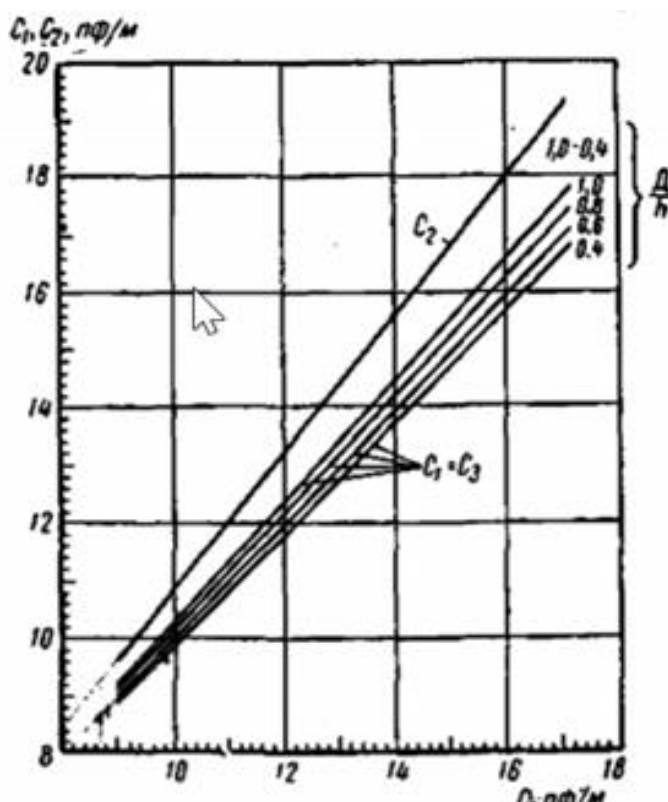
Рисунок 5.2 – Рабочие емкости линии электропередачи с горизонтальным расположением проводов: N — средняя высота провода над землей; D — расстояние между фазами; C_2 — емкость средней фазы; C — средняя емкость транспонированной линии без учета земле; C_1 = C_3 емкость крайних фаз трехфазной линии
