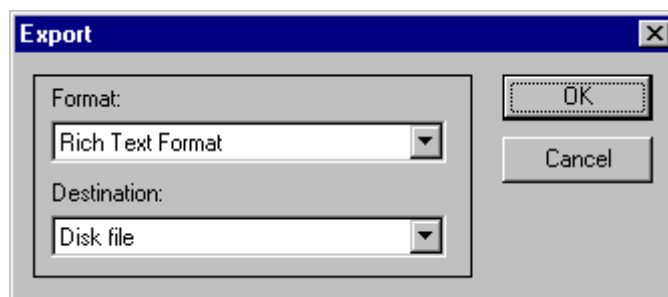
Рисунок 3.16 - Экспортный диалог
