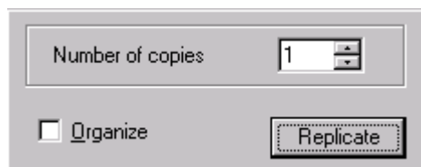
Рисунок 8.10 - Диалог копирования
