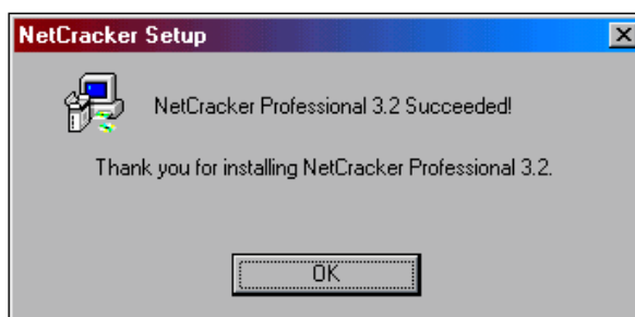
Рисунок 2.4 – Установка завершена
