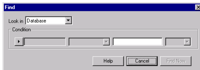
Рисунок 8.12 - Диалог Find
