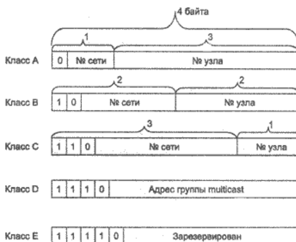
Рисунок 1.1 - Классы IP-адресов
