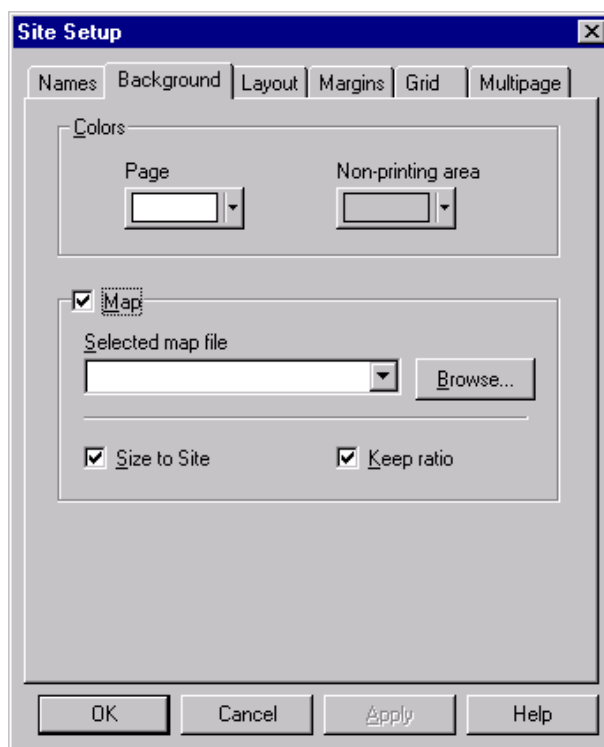
Рисунок 5.4- Диалог Установки
