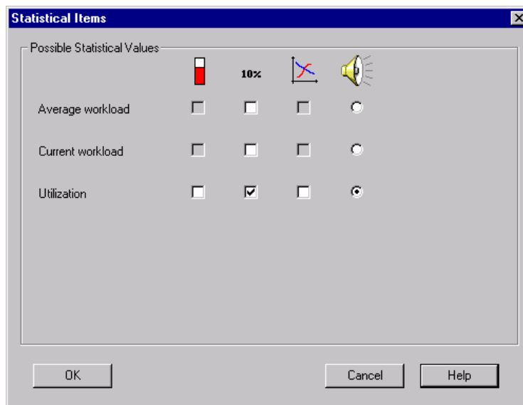
Рисунок 7.1 - Диалог статистики
