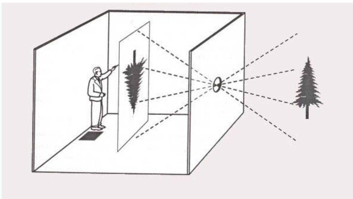
Камера-обскура
