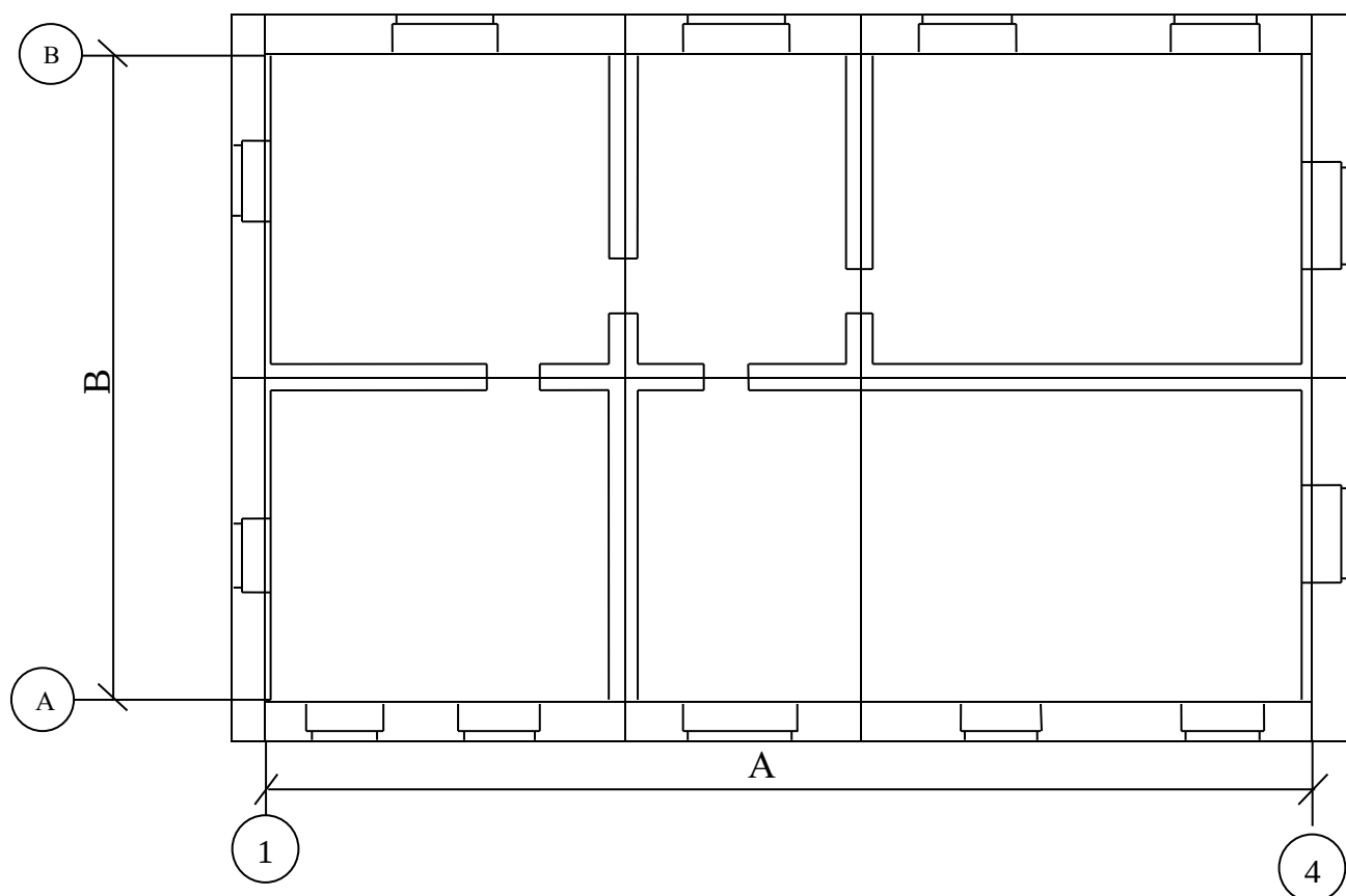
Рисунок 2.1 - Расчетная схема здания
