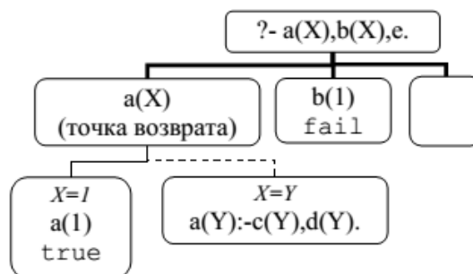
Рисунок 1.6 – Выполнение программы
