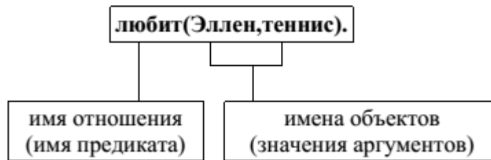
Рисунок 1.2 – Синтаксис Пролог
