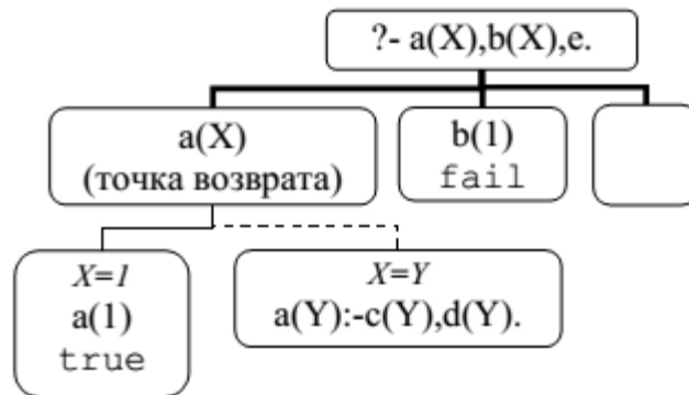
Рисунок 1.6 – Выполнение программы
