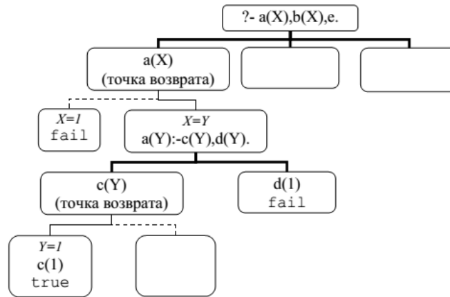
Рисунок 1.7 – Выполнение программы
