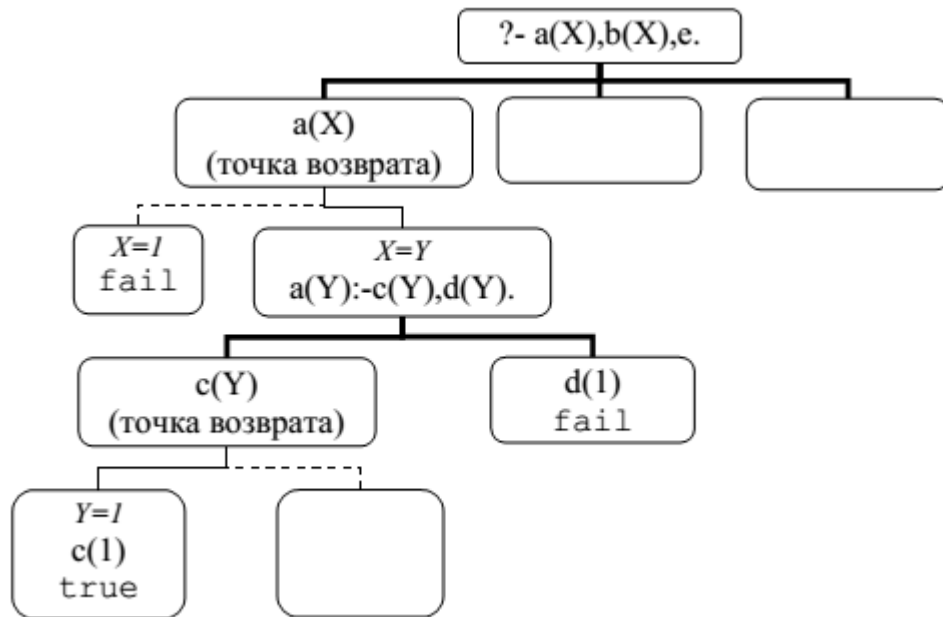
Рисунок 1.7 – Выполнение программы
