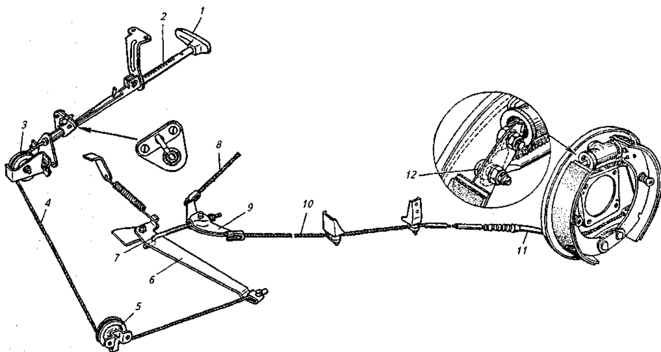
Рис. 25 Стояночный тормоз, действующий на задние колеса: 1 — рукоятка; 2 — рычаг; 3, 5 — ролики троса; 4 — передний трос; 6 — промежуточный рычаг; 7 — стержень; 8, 10 — тросы привода тормозных механизмов; 9 — уравниватель тормоза; 11 — трубка; 12 — эксцентриковая ось разжимного рычага
