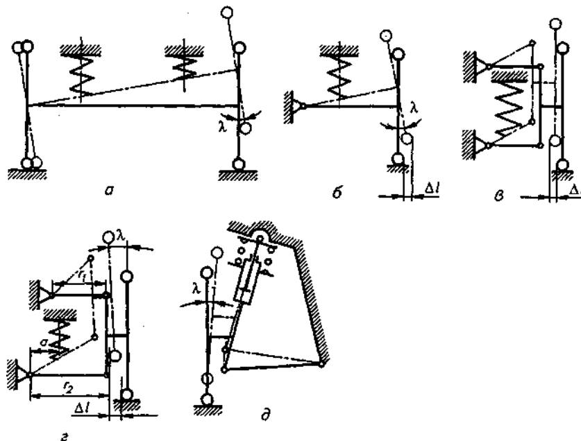
независимая рычажно-телескопическая
