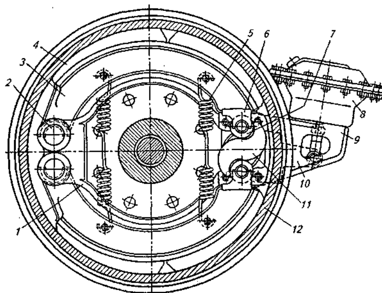
Рис. 1. Барабанный тормозной механизм: 1 — суппорт; 2 — опора колодки; 3 — колодка; 4 — фрикционная накладка; 5 — оттяжная пружина; 6 — опора ролика; 7 — ролик; 8 — тормозная камера; 9 — кронштейн тормозной камеры; 10 — регулировочный рычаг; 11 — разжимной кулак; 12 — тормозной барабан.
