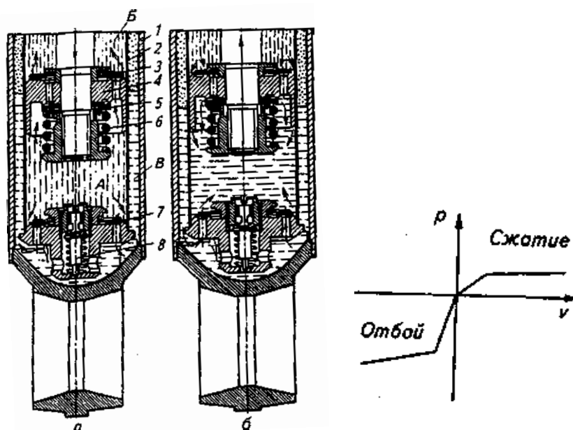
Рис. 15. Схема работы амортизатора: а – сжатие рессоры; б – отбой рессоры; в – характеристики амортизатора; А, Б, В – полости; 1 – рабочий цилиндр; 2 – корпус резервуара; 3 – перепускной клапан; 4 – поршень; 5 – клапан отбоя; 6 – пружина; 7 – всасывающий клапан; 8 – разгрузочный клапан
