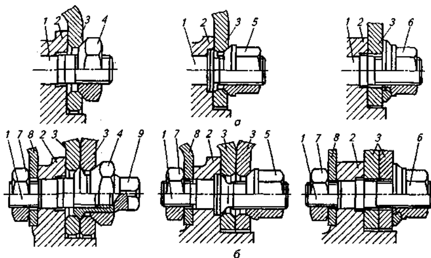
Рис. 10. Крепление дисковых колес грузовых автомобилей: а — одинарных; б — двойных; 1 — шпилька; 2 — ступица; 3 — диск; 4 — гайка крепления наружного диска; 5 — гайка типа ДИН; 6 — гайка с завальцованной шайбой; 7 — гайка крепления тормозного барабана; 8 — тормозной барабан; 9 — гайка крепления внутреннего диска
