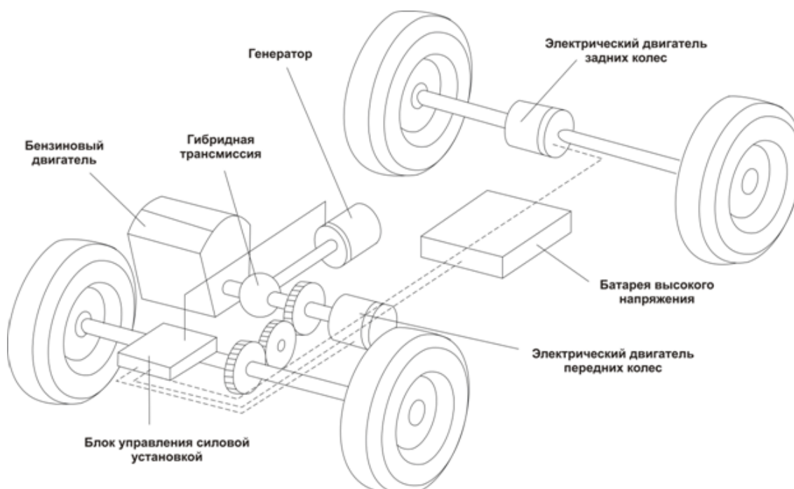
Рис. 5. Принципиальная схема последовательно-параллельной гибридной силовой установки
