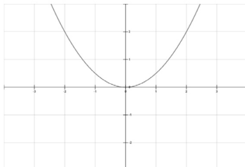
Рисунок 1 – Функция y = x^2
