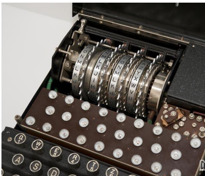
а) четыре последовательно соединённых ротора
