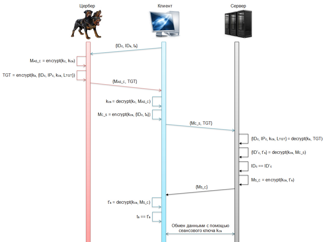
Рис.2. Проверка сервером S подлинности клиента С
