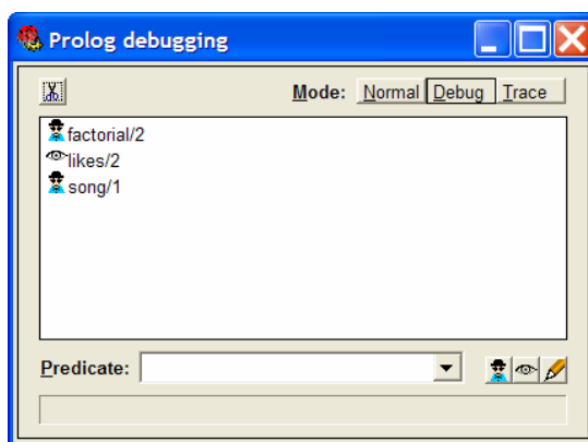
Рисунок 1.5 – Режим трассировки
