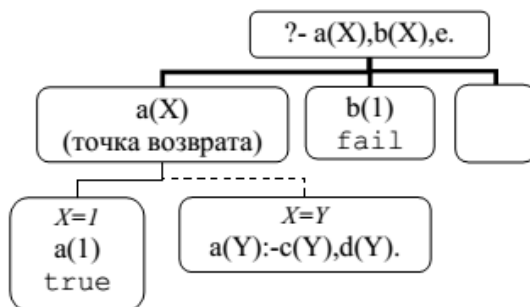
Рисунок 1.6 – Выполнение программы
