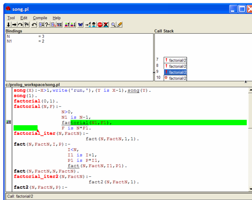
Рисунок 1.8 – Результат трассировки
