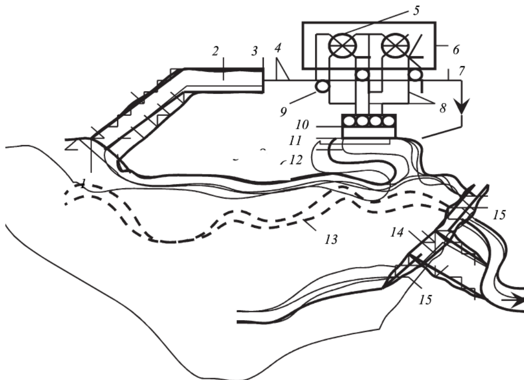
Рисунок 4.2 – Схема оборотного водоснабжения с прудом-охладителем:
