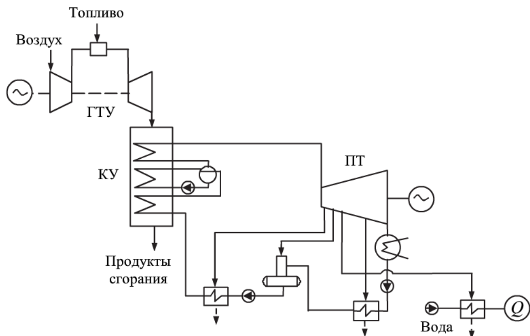
Рисунок 3.3 – Принципиальная тепловая схема ПГУ с КУ:
