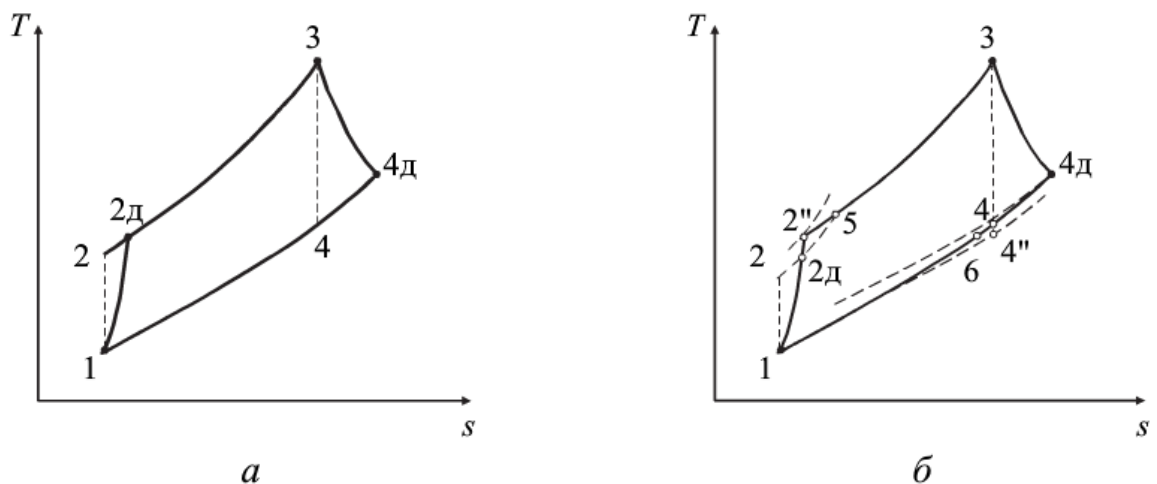
Рисунок 2.2 – Действительный цикл ГТУ без регенерации (а) и с регенерацией (б) при изобарном подводе теплоты в Т, s-диаграмме
