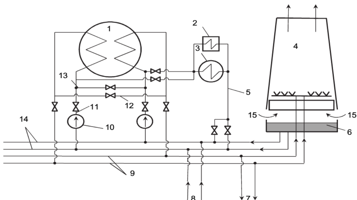
Рисунок 4.3 – Схема оборотного водоснабжения с градирней:
