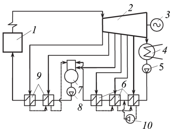
Рисунок 1.4 – Схема паросиловой установки с регенеративным подогревом воды:
