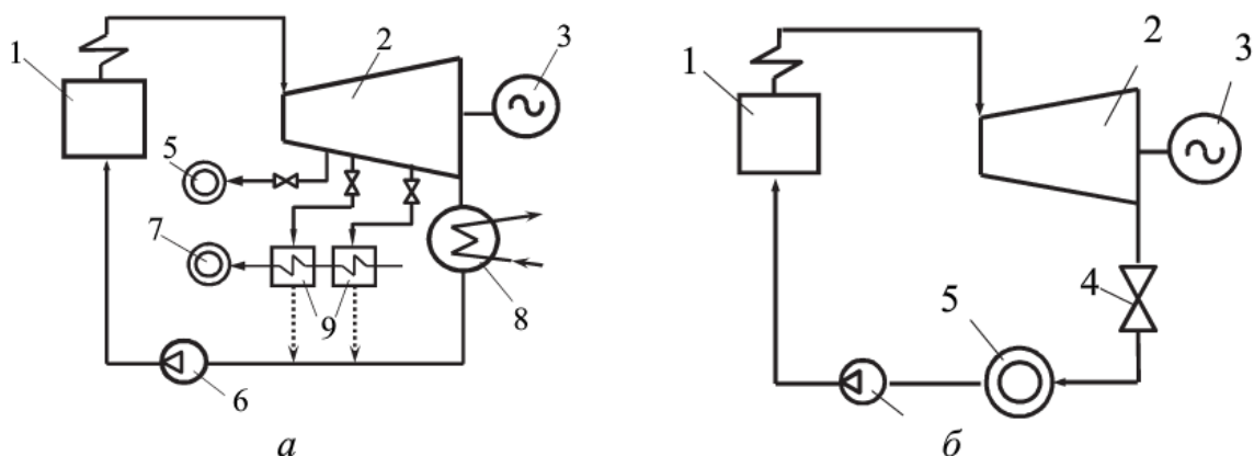
Рисунок 1.5 – Схема паросиловой установки с теплофикацией:
