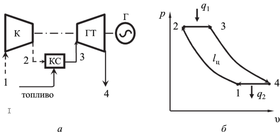
Рисунок 2.1 – Схема (а) идеальный цикл с изобарным подводом теплоты, (б) простейшей ГТУ:
