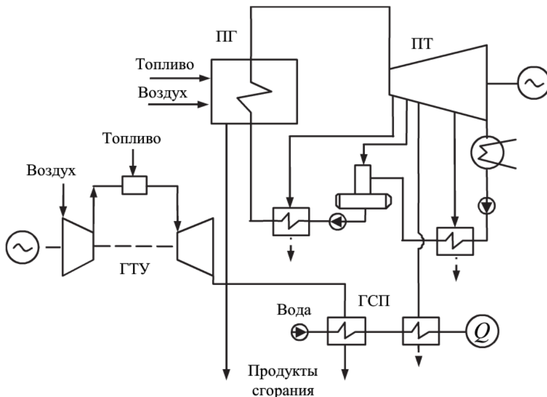
Рисунок 3.5 – Принципиальная тепловая схема ПГУ с ГСП:
