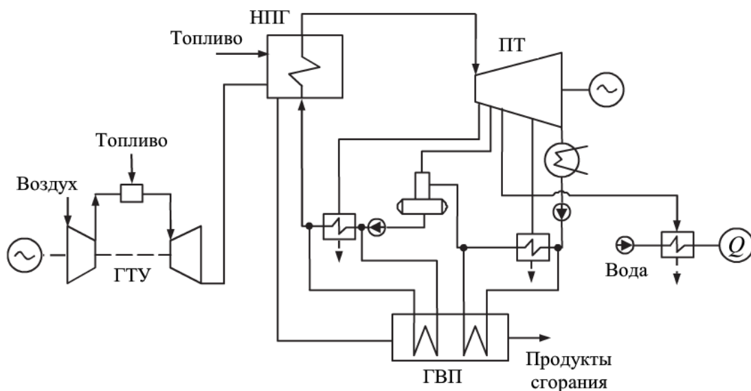
Рисунок 3.2 – Принципиальная тепловая схема ПГУ с НПП:
