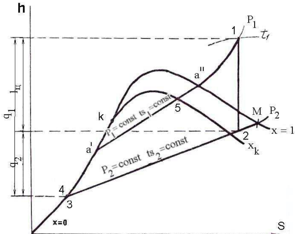
Рисунок 8.3 – h - s диаграмма цикла Ренкина
