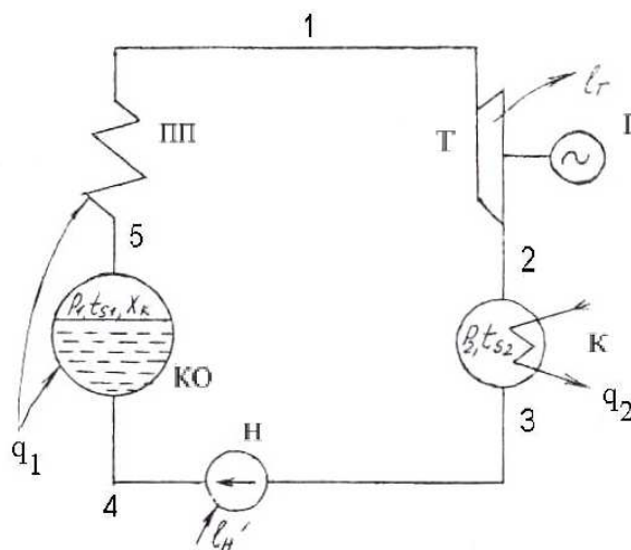
Рисунок 8.1 – Схема паросиловой установки, работающей по циклу Ренкина
