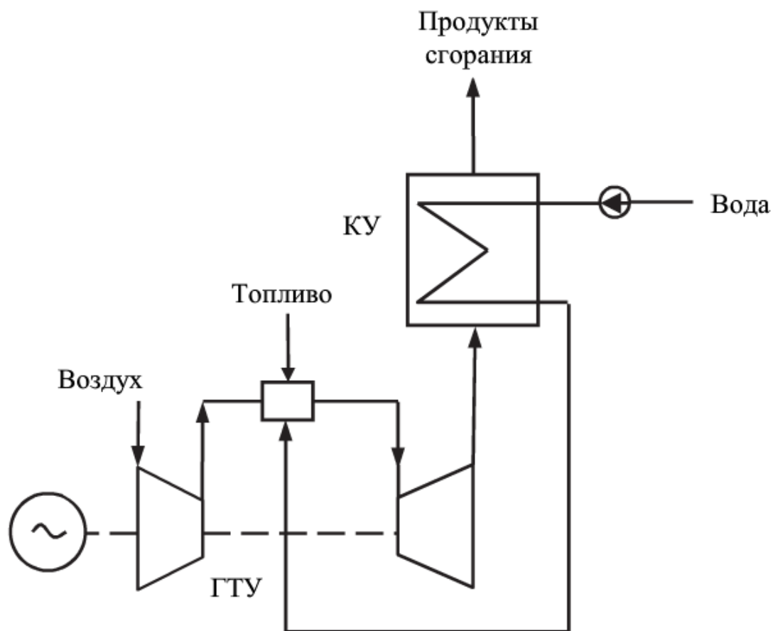
Рисунок 3.6 – Принципиальная тепловая схема со впрыском пара:
