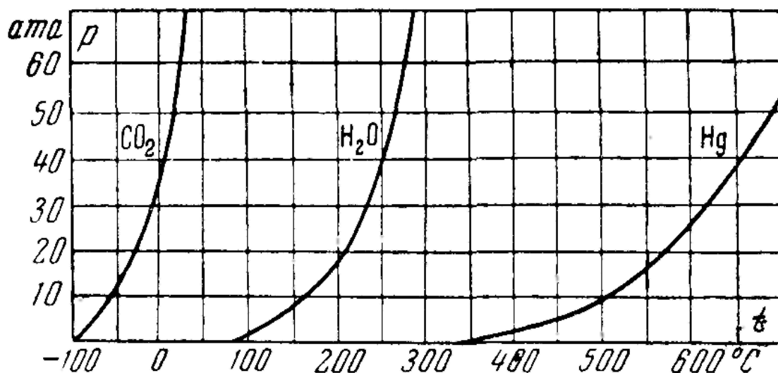
Рисунок 6.1 – Кривые зависимости между давлением и температурой кипения
