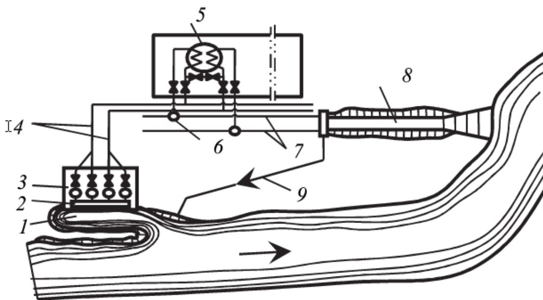
Рисунок 4.1 – Система прямоточного технического водоснабжения:
