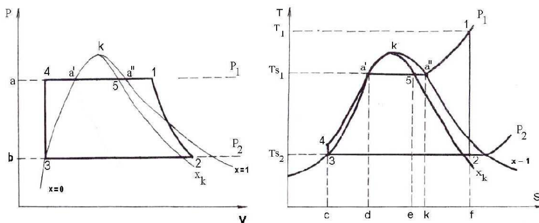
Рисунок 8.2 – PV и TS-диаграммы цикла Ренкина
