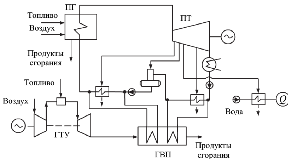
Рисунок 3.4 – Принципиальная тепловая схема ПГУ с ГВП:
