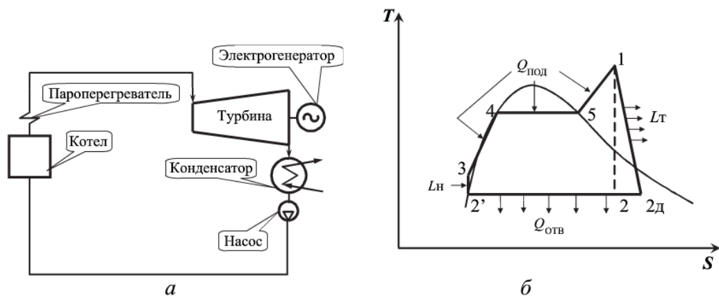
Рисунок 1.2 – ТЭС, работающая по циклу Ренкина:
