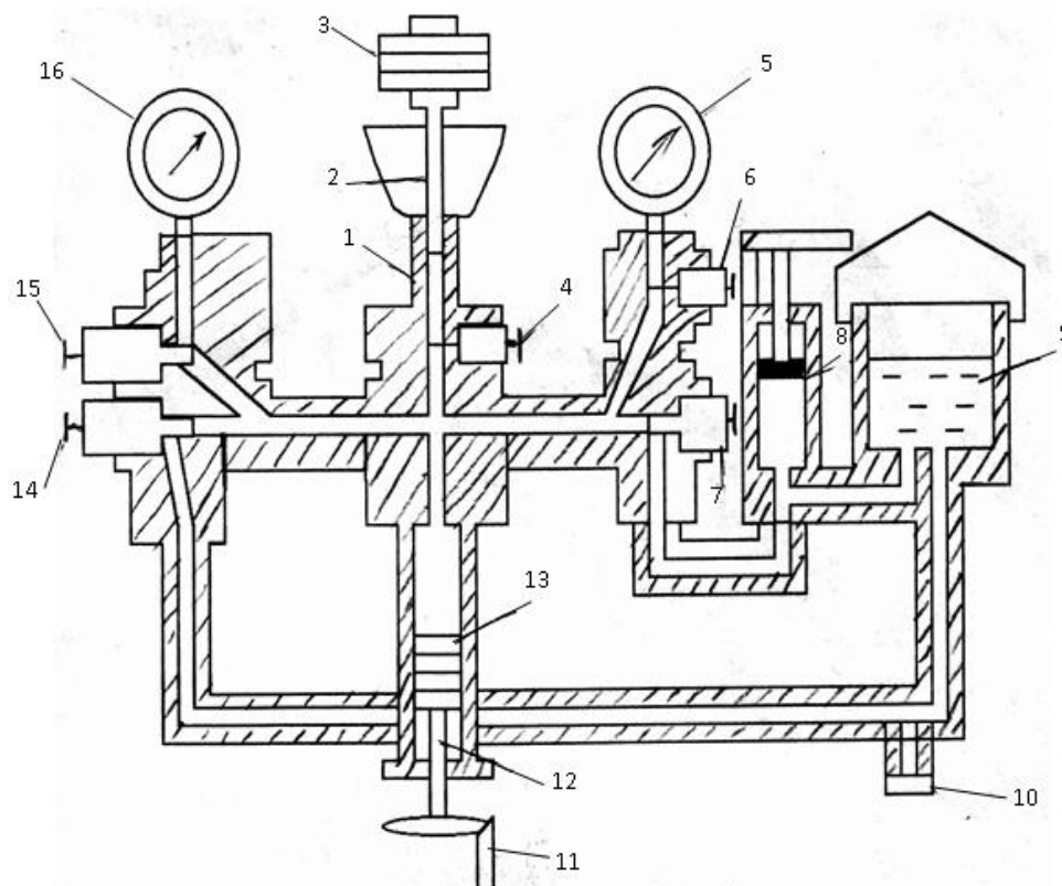
Рисунок 3 – Схема грузопоршневого манометра
