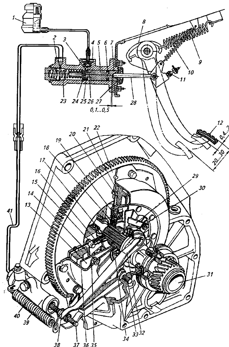
Рис. 7. Сцепление и привод сцепления автомобиля ВАЗ-21213: 1 — бачок для тормозной жидкости; 2— главный гидроцилиндр; 3— компенсационное отверстие; 4—штуцер; 5, 7—поршни; 6, 25—уплотняющие манжеты; 8—крючок; 9— пружина сервопривода; 10, 40—оттяжные пружины; 11— винт (ограничитель хода педали); 12—педаль; 13 — диафрагменная нажимная пружина; 14— опорная заклепка; 15— ступенчатая заклепка; 16— наружная пластина ведомого диска; 17— ступица ведомого диска; 18—фланец ступицы; 19—демпферная пружина; 20— нажимной диск; 21— ведомый диск; 22— маховик; 23 — пружина; 24— перепускное отверстие; 26— впускное отверстие; 27—стопорное кольцо; 28, 37— толкатели; 29— планка; 30— выжимной подшипник; 31 — вал сцепления; 32— вилка выключения сцепления; 33— шаровая опора; 34— упорный фланец; 35— опорное кольцо диафрагменной пружины; 36— кожух; 38— регулировочная гайка; 39— рабочий гидроцилиндр; 41 — трубопровод
