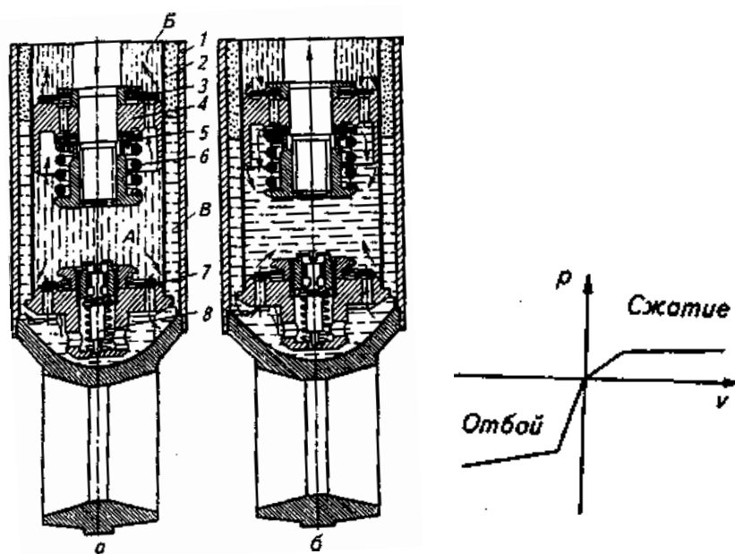
Рис. 15. Схема работы амортизатора: а — сжатие рессоры; б — отбой рессоры; в — характеристики амортизатора; А, Б, В — полости; 1 — рабочий цилиндр; 2 —
