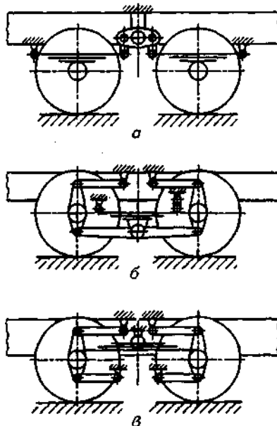
Рис. 14. Схемы балансирных подвесок: а — четырехрессорная с балансиrom; б — двухрессорная с жесткой балансирной балкой; в — с балансирными рессорами и реактивными штангами
