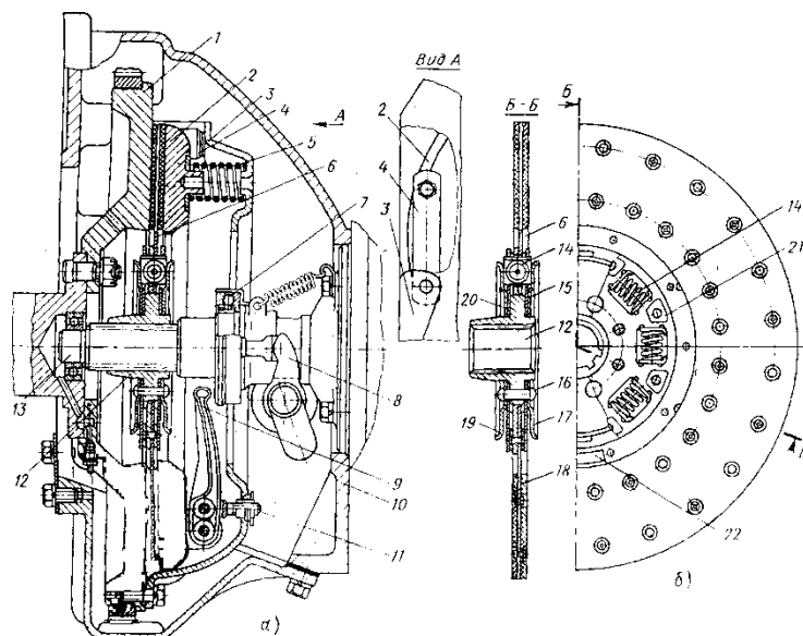
Рис. 5. Сцепление автомобиля ЗИЛ-130: а – общий вид; б – ведомый диск.
