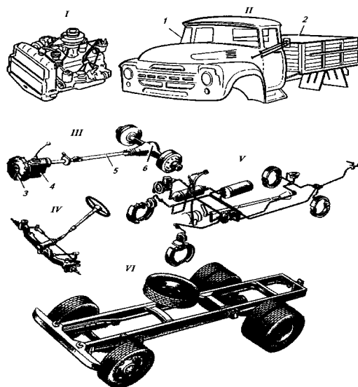
Рис. 13. Основные части автомобиля
