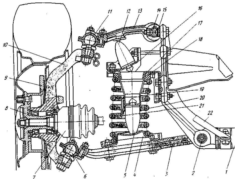
Рис. 22. Передняя подвеска легковой автомобиля ВАЗ-2121 «Нива»: 1 — поперечина; 2 — ось нижнего рычага; 3 — нижний рычаг; 4 и 17 — соответственно нижняя и верхняя опорные чашки пружины; 5 — буфер сжатия; 6 и 11 — соответственно нижний и верхний шаровые шарниры; 7 — наружный шарнир привода переднего колеса; 8 — ступица; 9 — тормозной диск; 10 — поворотный кулак; 12 — буфер отдачи; 13 — верхний рычаг; 14 — ось верхнего рычага; 15 — регулировочные прокладки; 16 — кронштейн; 18 — виброшумоизолирующая прокладка; 19 — опора; 20 — пружина; 21 — упор; 22 — растяжка
