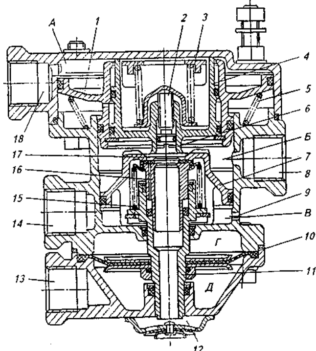
Рис. 18. Клапан тормозами двухприводом: полости
