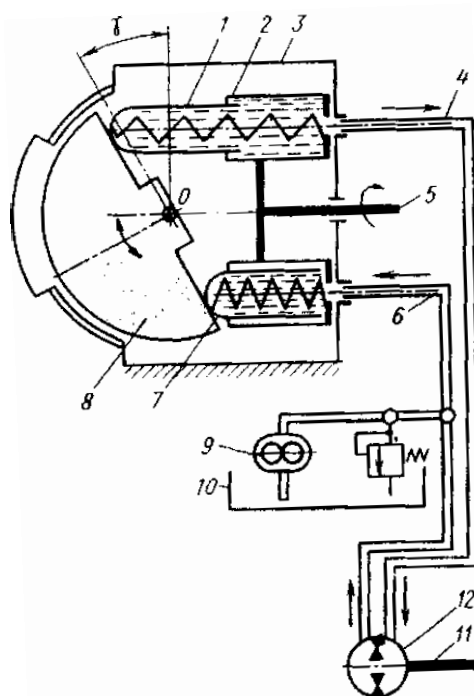
Рис. 6. Схема передач
