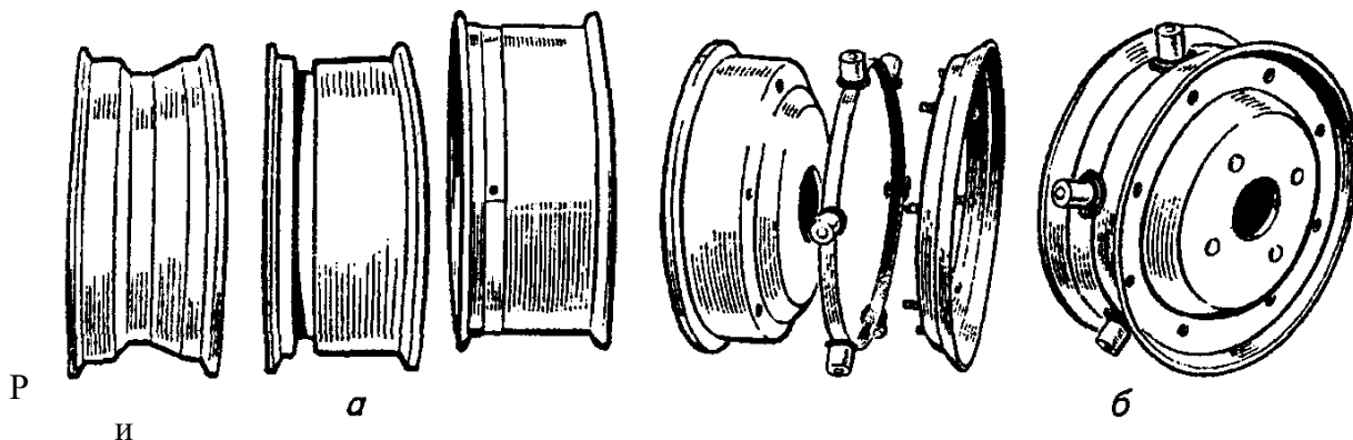
с. 3. Ободья для безопасных шин ТМТ: а — плоский обод, монтажный ручей которого закрыт пластмассовой лентой; б — разборный обод, снабженный капсулами со специальной жидкостью
