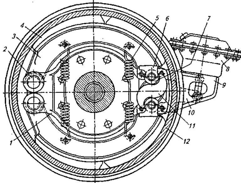
Рис. 1. Барабанный
