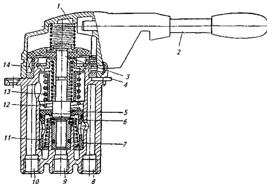
Рис. 19. Кран управления стояночным тормозом: 1, 11, 12, 13 — пружины; 2 — рукоятка; 3 — шток; 4 — фиксатор; 5 — седло; 6 — клапан; 7 — поршень; 8, 9, 10 — выводы; 14 — кулачки
