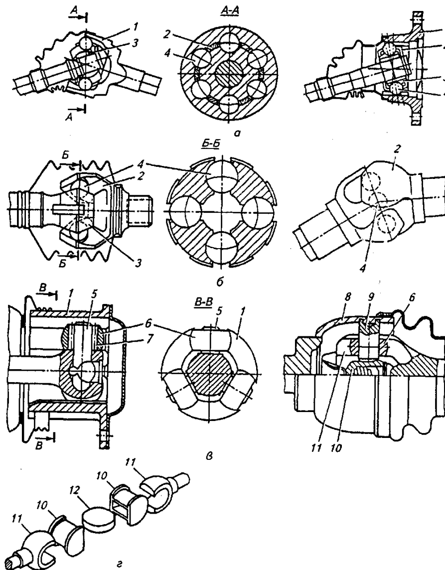
Рис. 3. Синхронные шарниры: а - с шестью шариками; б - с пятью и четырьмя шариками; в - трехшпиковые с роликами; г - дисковые; 1 - корпус; 2 - сепаратор; 3 - обойма; 4 - шарик; 5 - трехшпиковая крестовина; 6 - ролик; 7 - игла; 8 - чашка; 9 - шип; 10 - центрирующее устройство; 11 - вилка, 12 - диск
