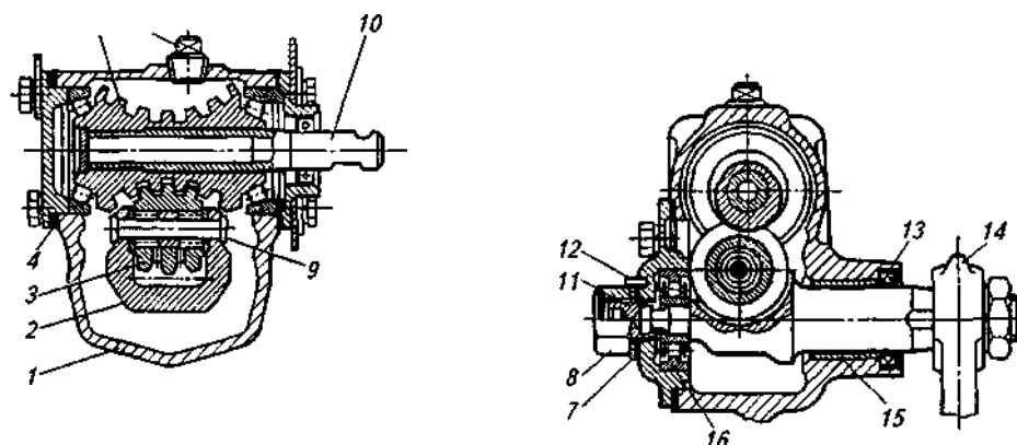
Рис. 2. Рулевой механизм типа червяк — ролик: 1 — картер механизма; 2— вал сошки; 3 — трехгребневый ролик; 4— прокладка; 5— червяк; 6 —пробка; 7—стопорная шайба; 8— колпачковая гайка; 9 —ось ролика; 10— вал руля; 11 — регулировочный винт; 12— стопорный штифт; 13 — сальник; 14— рулевая сошка; 15— бронзовая втулка; 16— роликовый подшипник.
