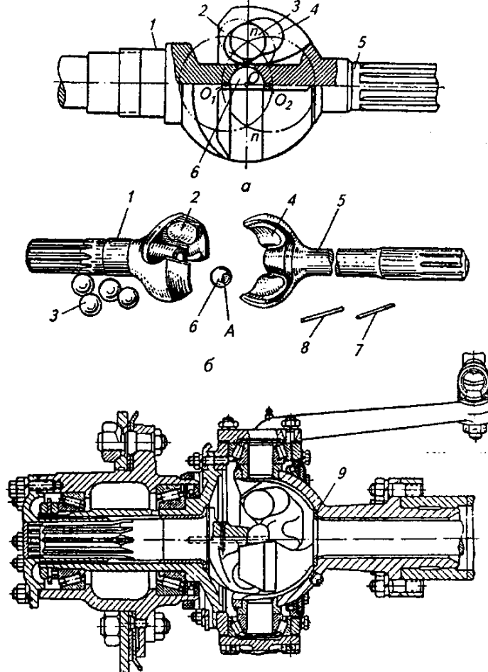
Рис. 4. Шариковый равных
