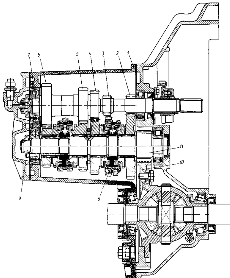
10. Коробка передач
