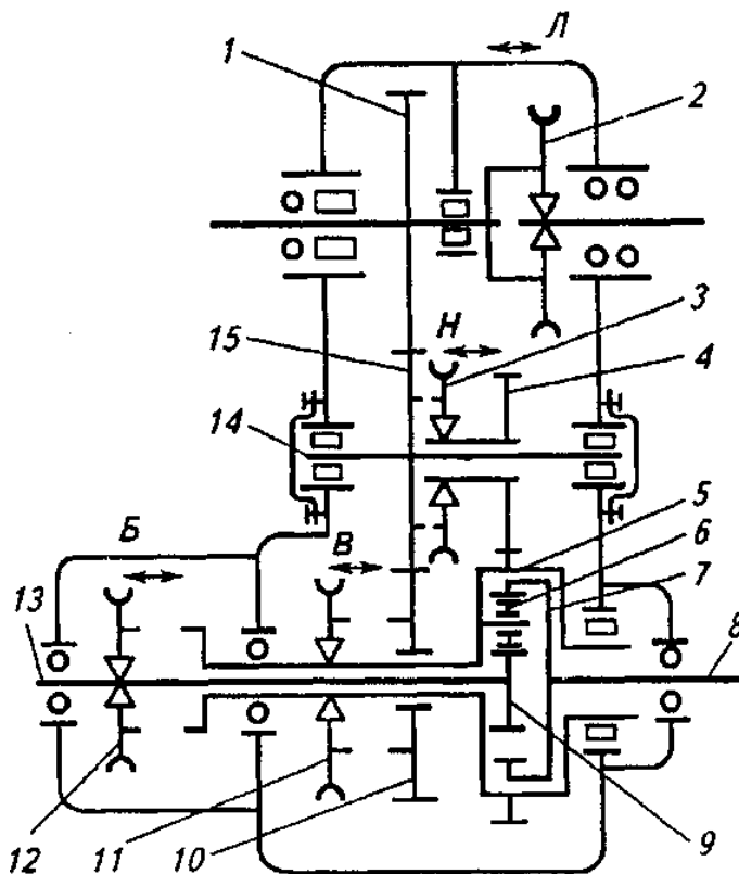
Рис. 14. схема раздаточной автомобиля КамАЗ-
