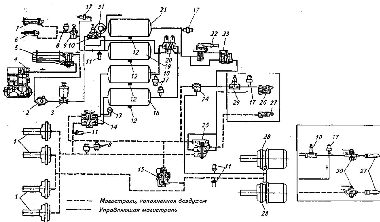
Рис. 11. Схема пневмопривода автомобиля КАЗ-4540: 1 — тормозные камеры передних колес; 2 — регулятор давления; 3 — предохранитель от заморозания; 4 — компрессор; 5 — влагоотделитель; 6 — пневмоцилиндр привода рычага останова двигателя; 7 — пневмоцилиндр привода механизмов вспомогательного тормоза; 8, 17 — пневмоэлектрические датчики; 9 — пневматический кран вспомогательного тормоза; 10 — одинарный перепускной защитный клапан (без обратного клапана); 11 — клапаны контрольного вывода; 12 — краны слива конденсата; 13 — двухстрелочный манометр; 14 — двухсекционный тормозной кран; 15 — регулятор тормозных сил; 16 — воздушный баллон контура рабочего тормоза переднего моста; 18 — воздушный баллон контура рабочего тормоза заднего моста; 19 — воздушный баллон прочих потребителей; 20 — тройной защитный клапан; 21 — воздушный баллон контура стояночного и вспомогательного тормозов; 22 — кран стояночного тормоза; 23 — ускорительный клапан; 24 — двухмагистральный клапан; 25 — клапан управления тормозами прицепа с двухпроводным приводом; 26 — автоматическая соединительная головка; 27 — соединительная головка типа «Палм»; 28 — тормозная камера задних колес с пружинным энергоаккумулятором; 29 — защитный одинарный клапан с обратным потоком; 30 — разобщительный кран; 31 — редукционный клапан
