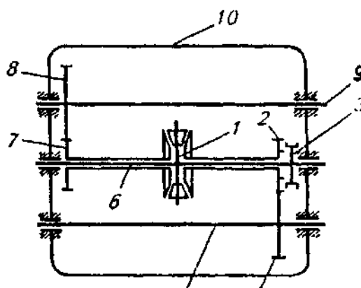
Рис. 9. Межосевой дифференциал: 1 — крестовина; 2, 4, 7, 8 — шестерни; 3 — муфта; 5 — вал привода среднего моста; 6 — ведущий вал межосевого дифференциала; 9 — вал привода заднего моста; 10 — корпус
