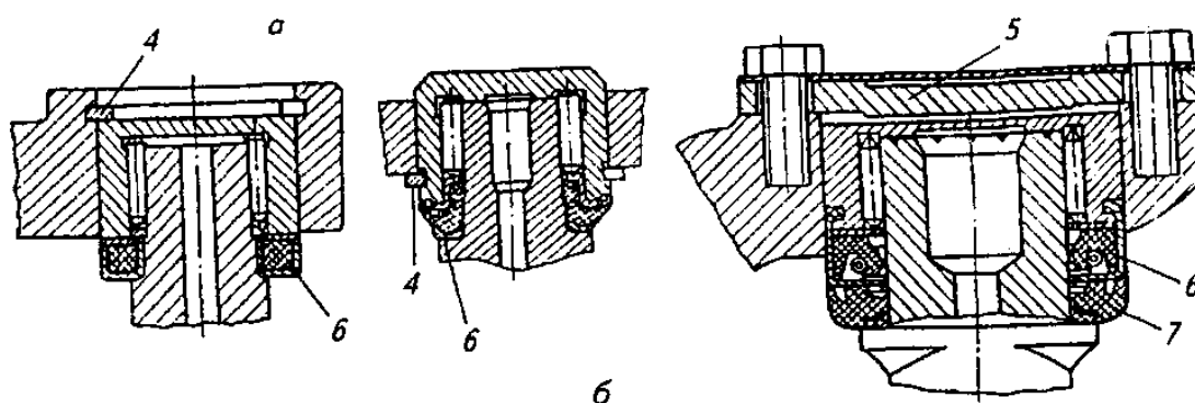
Рис. 12. Вилки игольчатых карданов неравных угловых скоростей: а —вилка игольчатого кардана; б— варианты крепления стакана и уплотнения игольчатого подшипника; 1 —проушина вилки; 2, 3— фланцы; 4 — стопорное кольцо; 5 — крышка; 6 — самоподжимной сальник; 7— резиновый торцевой сальник
