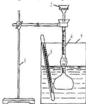
1 - штатив, 2 – воронка, 3 – термометр, 4 –объёмомер, 5 – стеклянный сосуд Рисунок 1 - Прибор для определения истинной плотности
