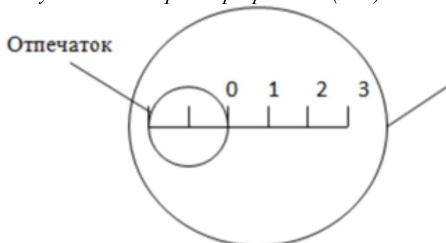
Рисунок 2.2 - Твердомер Бринелля (ТШ)
