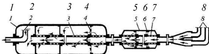
Рис. 1. Схема глушителя отработавших газов:
