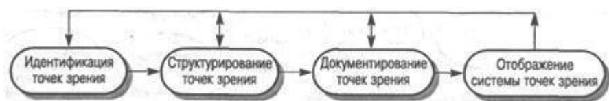
Рисунок 1.3 - Метод VORD
