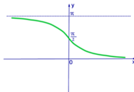
Рис.4 График функции y = \text{arcctg} x
