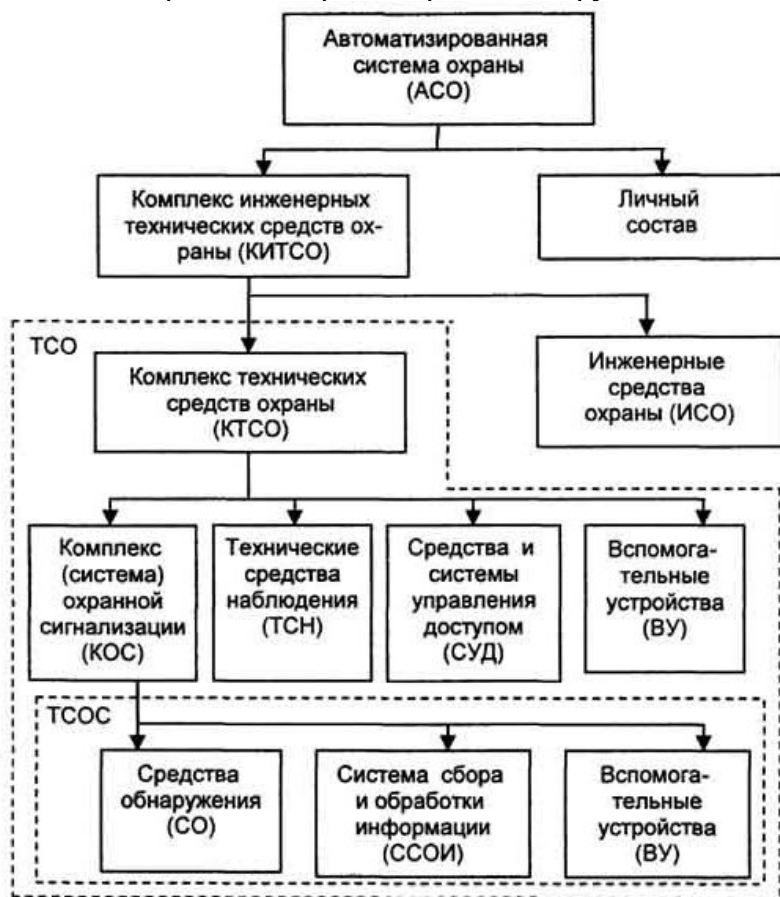
Рис. 1. Структура автоматизированной системы охраны
