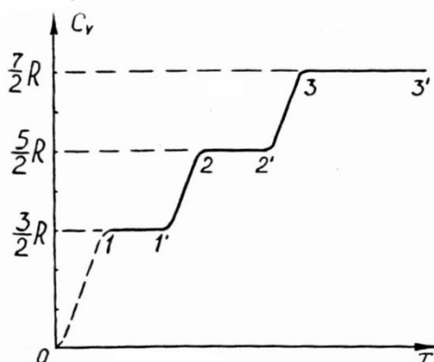
Рисунок 2 – Зависимость молярной теплоемкости от температуры газа
