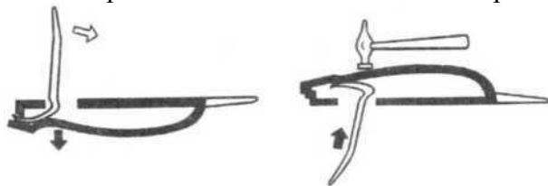
Рис. 6.2. Выколотка труднодоступных полостей
