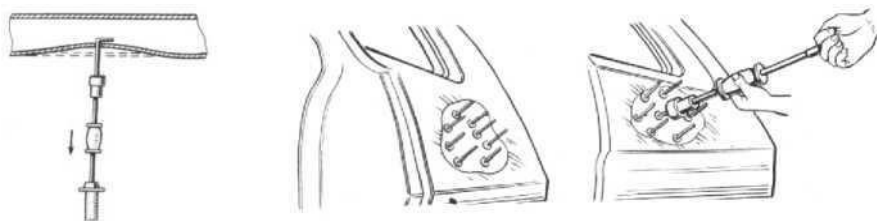
Рис. 6.3. Применение инерционного молотка
