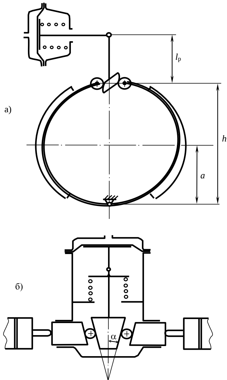
Рисунок 2.1 - Схемы тормозных механизмов: а – кулачковый; б - клиновой.
