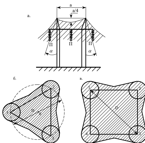
Рисунок 8.3 – Зоны защиты
