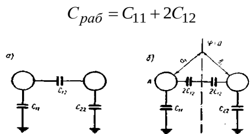
Рисунок 3.2 – Схема для расчета частичных емкостей двухпроводной линии: а — для расчета емкости линии; б — для расчета рабочей емкости провода
