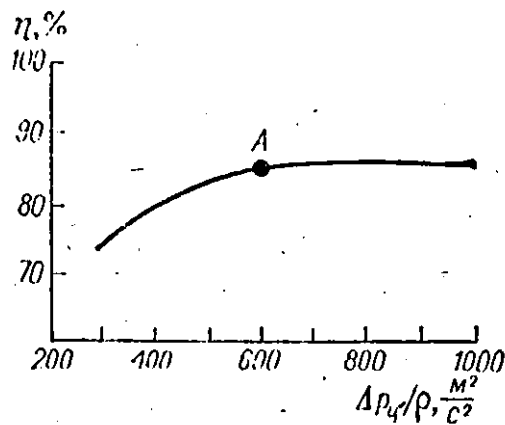
Рис. 3. Зависимость степени очистки п циклона от соотношения \Delta p_{\text{ц}}/\rho
