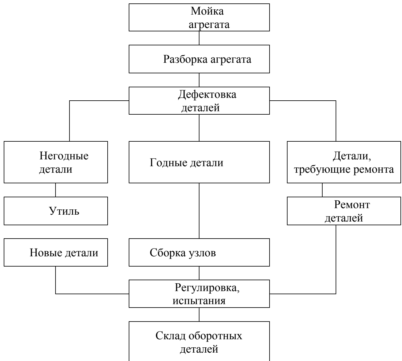
Рис. 4. Схема технологического процесса ремонта агрегатов в цехе (участке)
