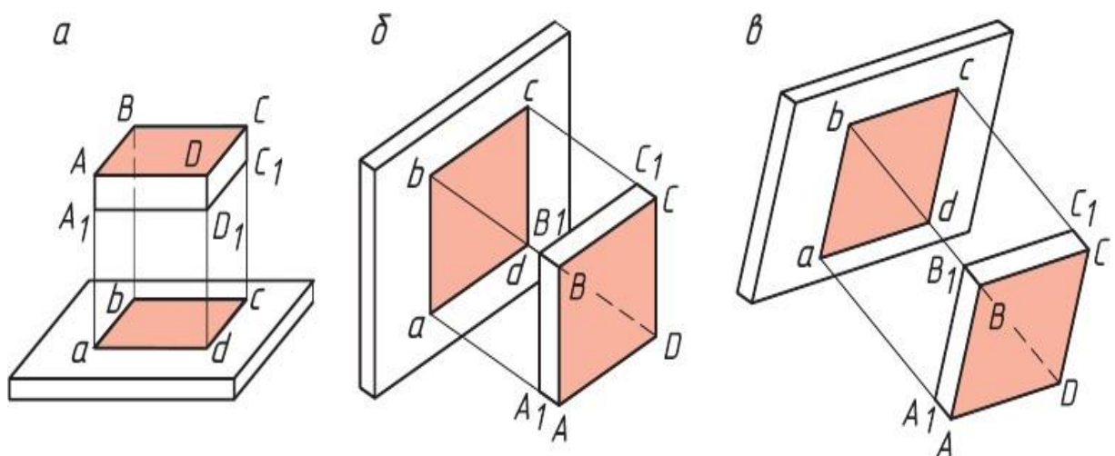
Рис. 41. Прямоугольное проецирование
