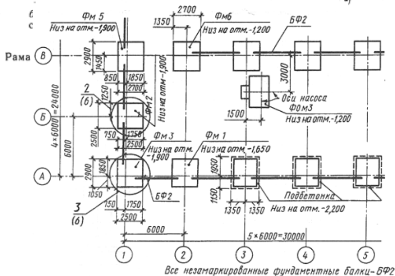
Схемы расположения колонн и балок (план и разрез 1-1) многоэтажного
