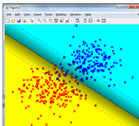
Рисунок 4.4 – Решение на обучающей выборке
