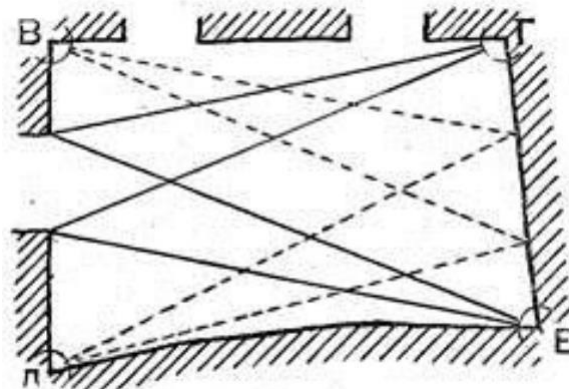
Рисунок 4а триангуляционная система обмер
