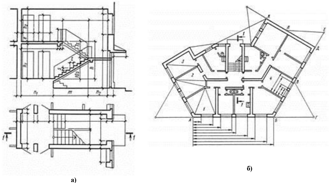
Рисунок 2 – Подготовки для обмеров а) лестничной клетки; б) плана здания.
