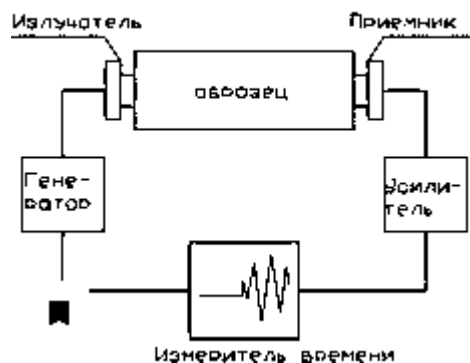
ПРИНЦИПИАЛЬНАЯ СХЕМА
