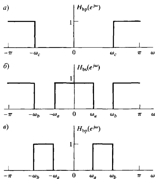
Рис. 1.2. Идеальные частотно-избирательные фильтры.
