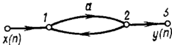
Рисунок 3. Пример невыхислимого направленного графа
