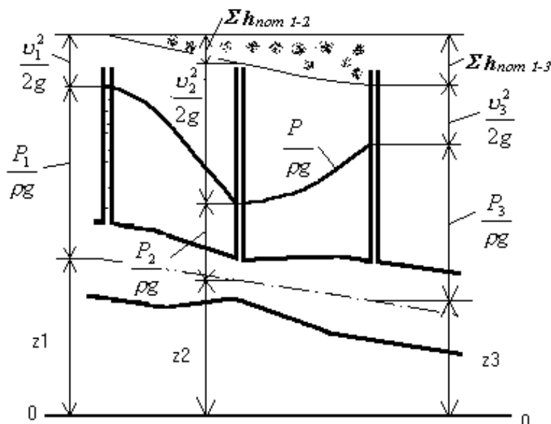
Рис. 1.6. 2. Графическая интерпретация закона Бернулли
