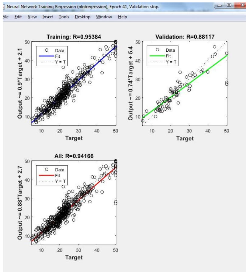
Рисунок 7.6 – Отношение данных (кружки) к получившимся моделям (линии)
