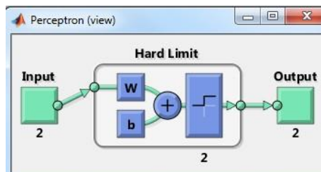
Рисунок 3.20 – Общая структура персептрона
