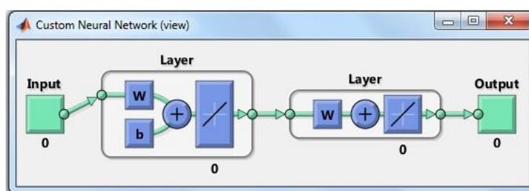
Рисунок 3.4 – Изначальная структура сети
