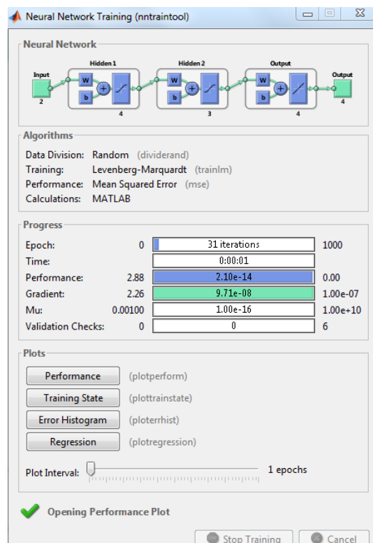
Рисунок 3.35 – Обучение сети, потребовалось 31 итерация
