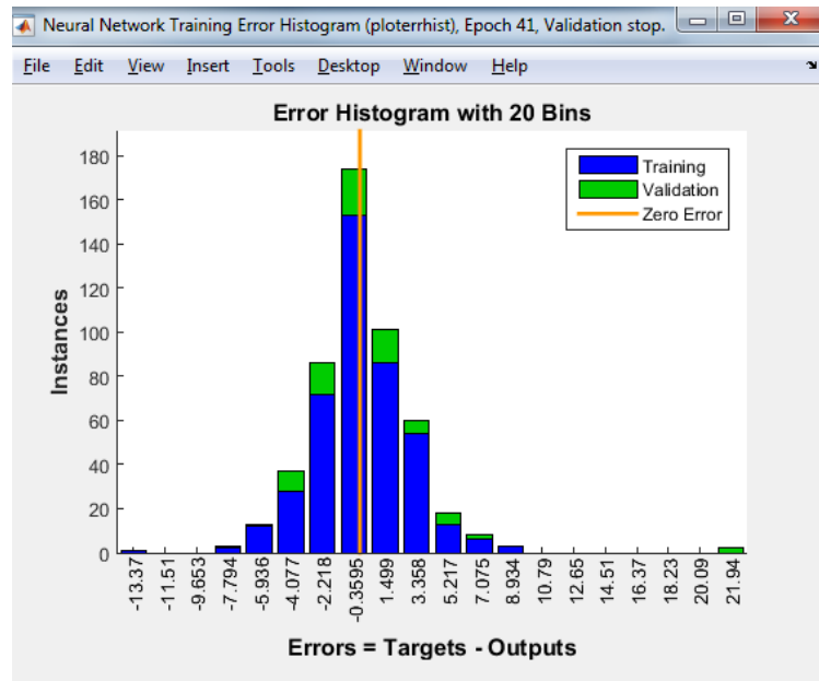
Рисунок 7.5 – Диаграмма распределения фактической ошибки при предсказании
