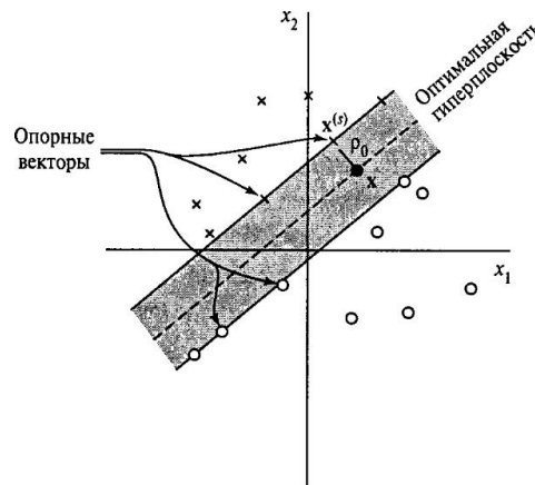
Рисунок 4.2 – Оптимальная гиперплоскость для линейно разделимых образов Данное
