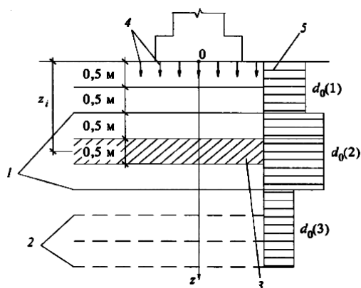
Рис. 3.7. Схема для расчета рассоления основания при вертикальной фильтрации 1 - границы слоев с различным содержанием гипса; 2 - границы расчетных слоев; 3 - расчетный слой; 4 - направление фильтрации; 5 - начальная эпюра относительного содержания гипса d_0(z)
