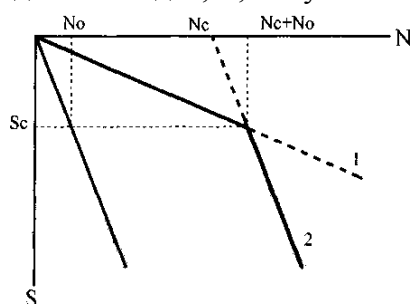
Рис. 3.14.- Схема этапов расчета нагружения сваи по формулам: 1 - (3.27); 2 - (3.29)
