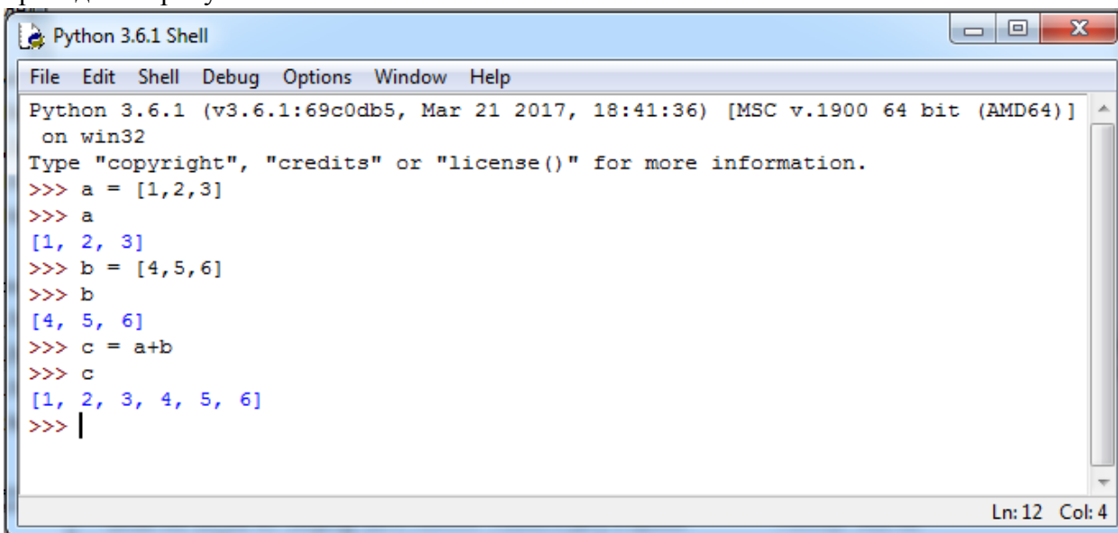
Рисунок – Интерактивный интерпретатор PythonShell. Пример работы со списками.
