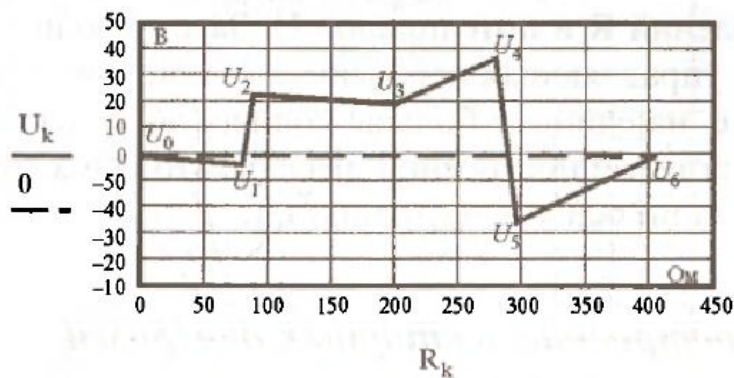
Рис. 3.5. Построение потенциальной диаграммы для цепи постоянного тока с двумя источниками ЭДС
