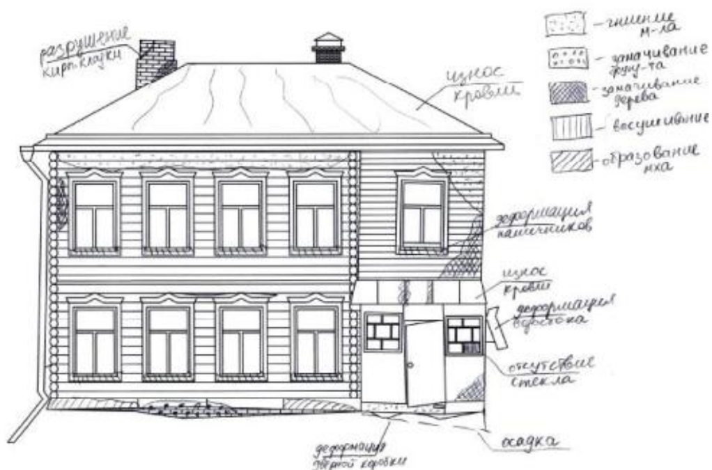
Рисунок 3 – Дефектная карта фасада
