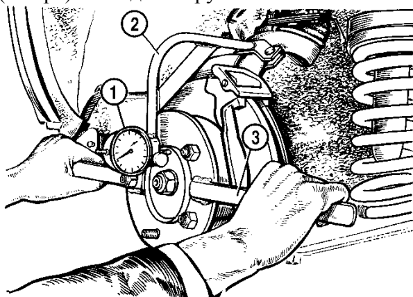
Рис. 4.1. Измерение зазора в ступичных подшипниках
