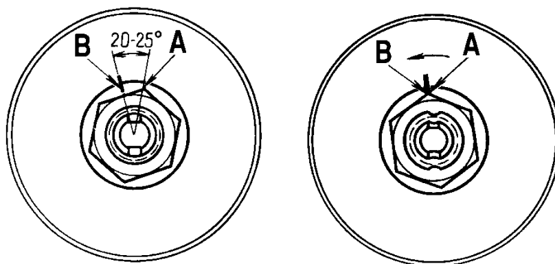
Рис. 4.2. Схема затяжки гайки ступицы
