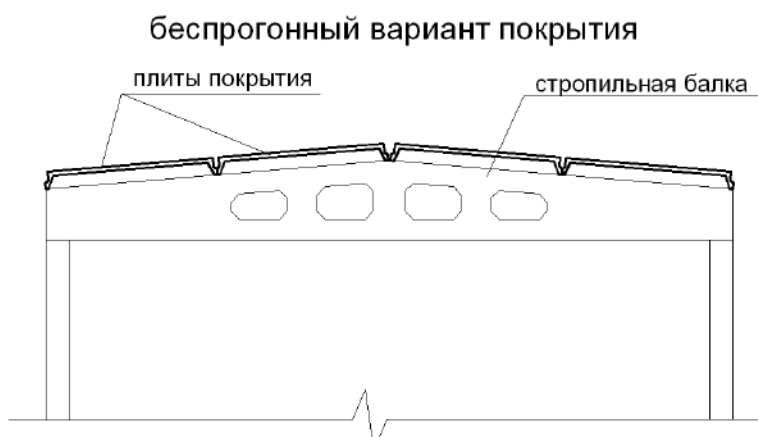
Рисунок 1–беспрогонный вариант покрытия
