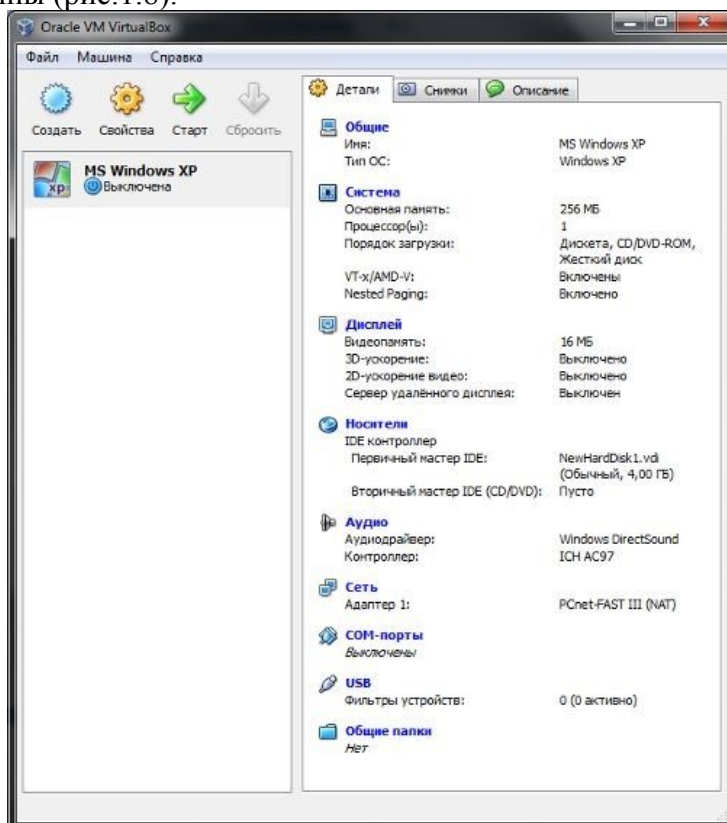
Рис. 1.8. Консоль управления виртуальных машин «Oracle VirtualBox»
