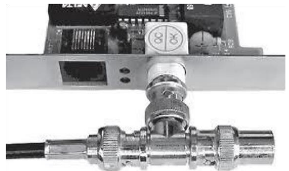
Рис. 2. Т-коннектор, присоединенный к сетевой карте
