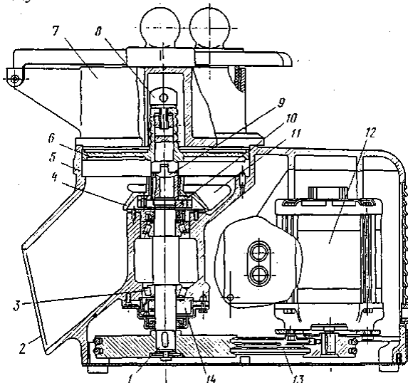
Рисунок 2.7 - Универсальная овощерезательная машина МРО 50-200
