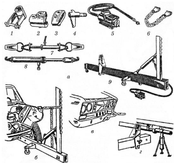
Рис.17.Приспособления для выполнения правки деформированного участка кузова:
