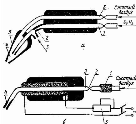
Рис.2. Схема горелок для сварки термопластов горячими газами:
