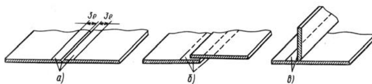
Рис.4.Подготовка кромок пайке латунным припоем: а – участки, зачищенные до металла; б и в – зачистка до чистого металла
