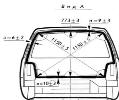
Рис.9.Размеры проемов и зазоры сопрягаемых деталей кузова автомобиля модели ВАЗ-
