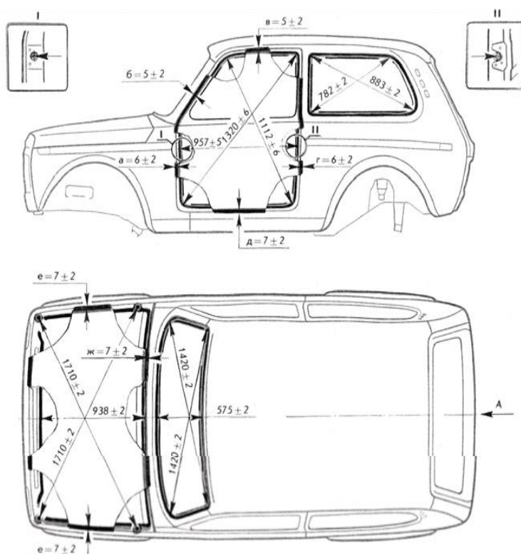
Рис.7.Размерыпроемовизорысопрягаемыхдеталейкузова автомобилямоделиВАЗ-2121
