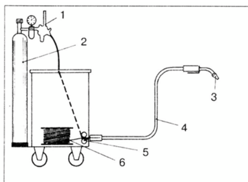
Рис. 10. Схема аппарата для сварки в среде защитного газа: 1 – редуктор; 2 – газовый баллон; 3 – горелка; 4 – направляющий шланг; 5 – механизм подачи проволоки; 6 – катушка с проволочным электродом
