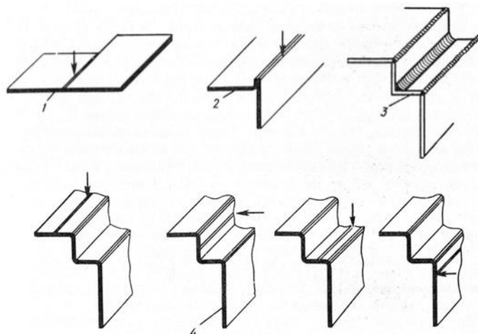
Рис. 6. Подготовка кромок тонких листов под сварку:
