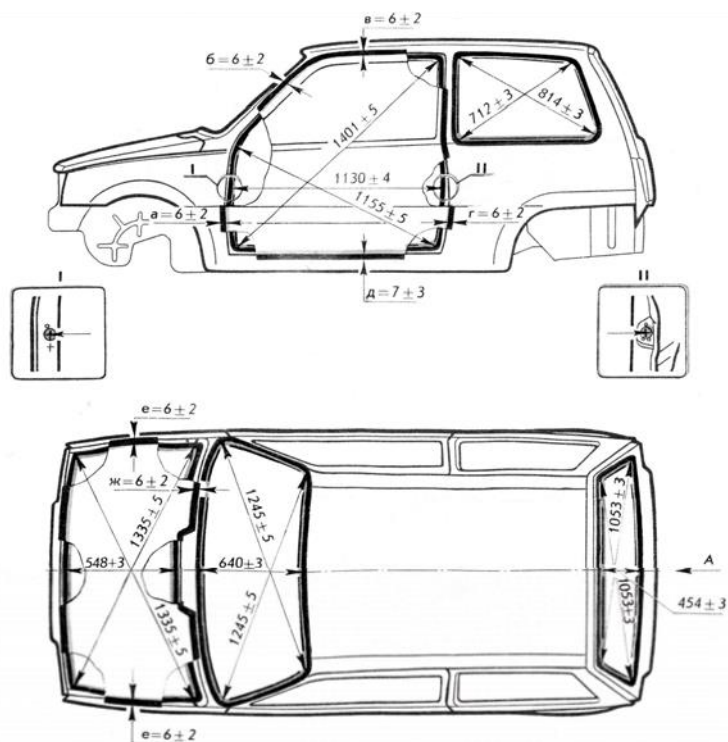
Рис.9.Размеры проемов и зазоры сопрягаемых деталей кузова автомобиля модели ВАЗ-
