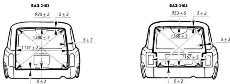
Рис.6.Размерыпроемовизорысопрягаемыхдеталейкузова автомобилеймоделейВАЗ-2101- 2107
