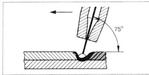
Рис. 11. Положение горелки при сварке в среде защитного газа
