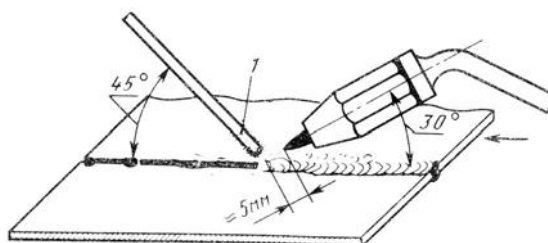
Рис.5.Расположение горелки и припоя при пайке латунным припоем: 1 – порошковый флюс, нанесенный на конец припоя или прутка, покрытый флюсом
