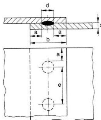
Рис.14. Геометрические параметры контактно-точечной сварки:
