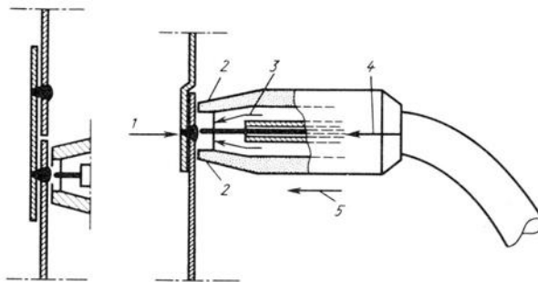
Рис. 12. Точечная сварка тонких листов, один из которых выполнен с накладной лентой, а другой с отбортовкой:
