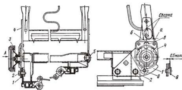
Рис. 2. Замена бесступенчатого механизма регулирования угла наклона спинки сиденья
