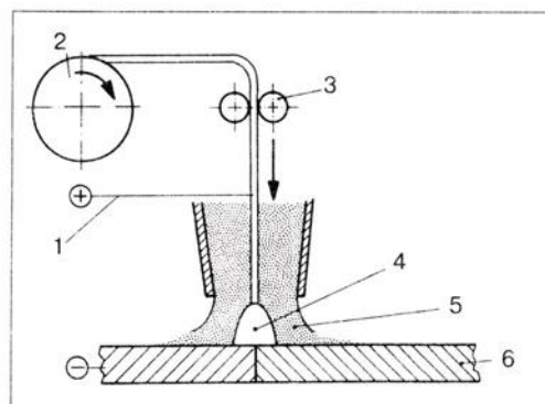
Рис.9. Схема процесса сварки в среде защитного газа: 1 – электрод; 2 – катушка проволочного электрода; 3 – механизм подачи проволочного электрода; 4 – электрическая дуга; 5 – защитный газ; 6 – деталь
