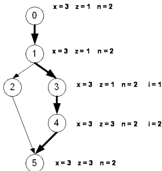
Рис. 3.1. Управляющий граф программы
