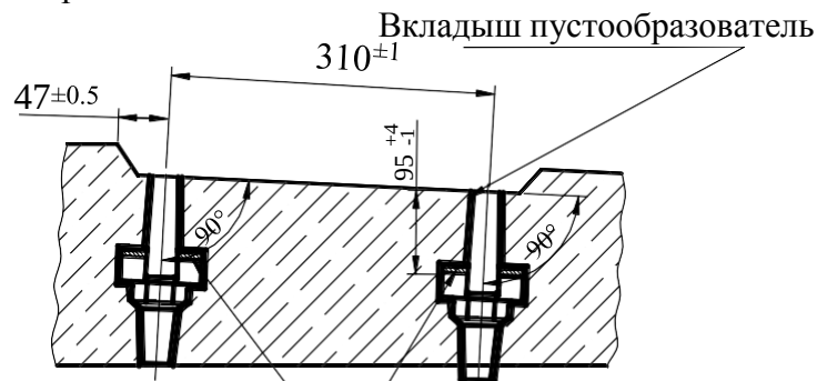
Рис. 7.3. Нормативная геометрическая модель подрельсовой части шпалы.
