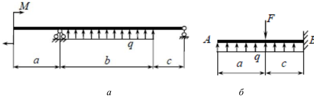
Рис. 3.1 Конструктивные схемы балок: a - двухопорной и б – консольной
