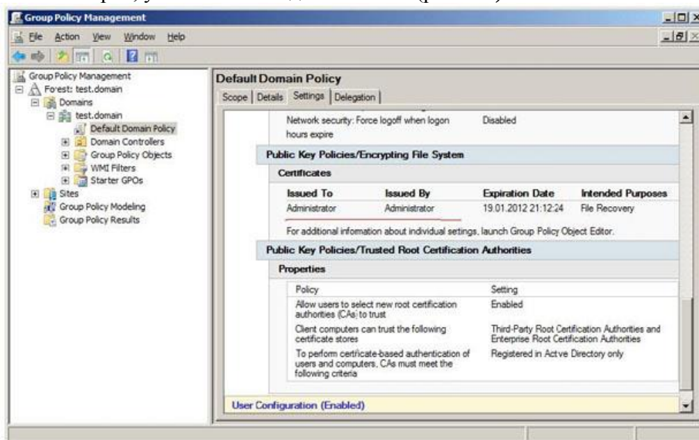
Рис. 7.3. Агент восстановления
