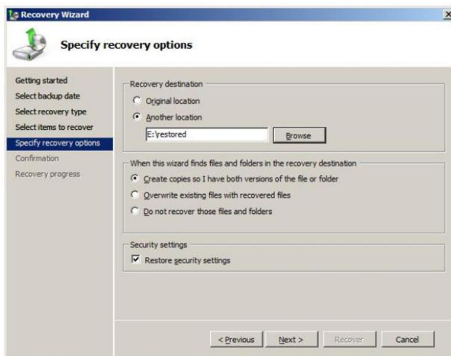
Рис. 9.8. Параметры восстановления
