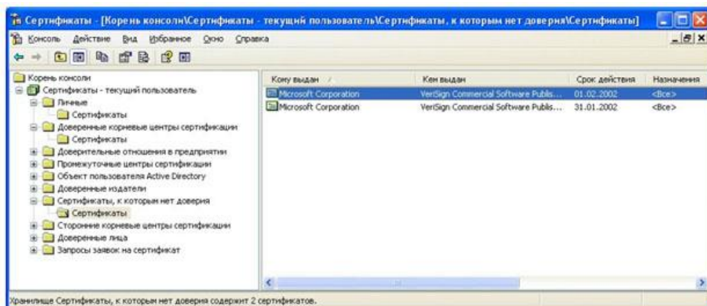
Рис. 8.4. Отзывные сертификаты
