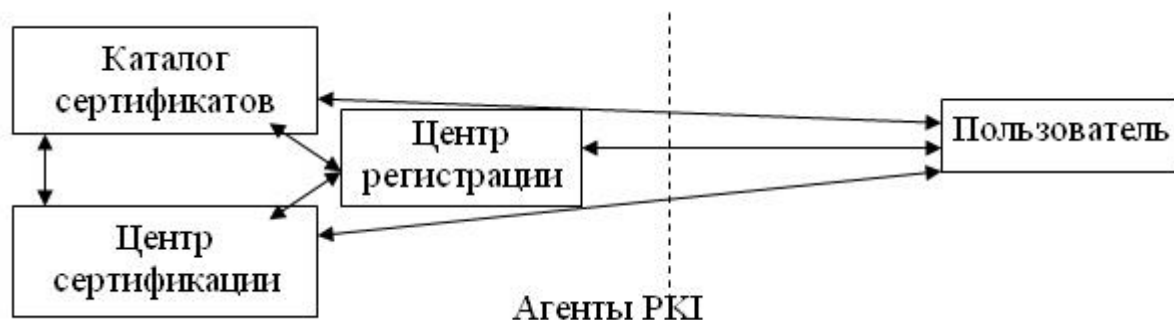
Рис. 2. Структура PKI
