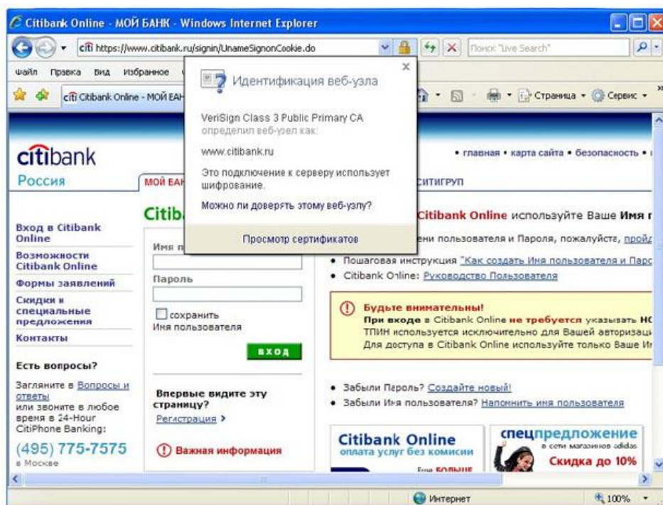
Рис. 8.1. Защищенное соединение
