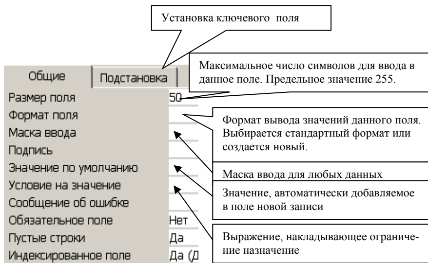
Рисунок 2. Свойства текстового поля
