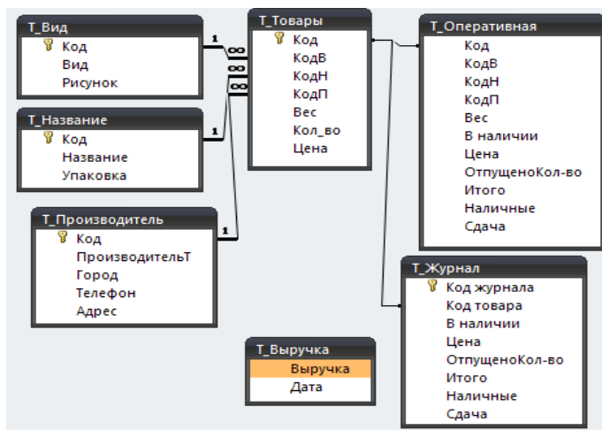
Рисунок 4. Пример схемы данных
