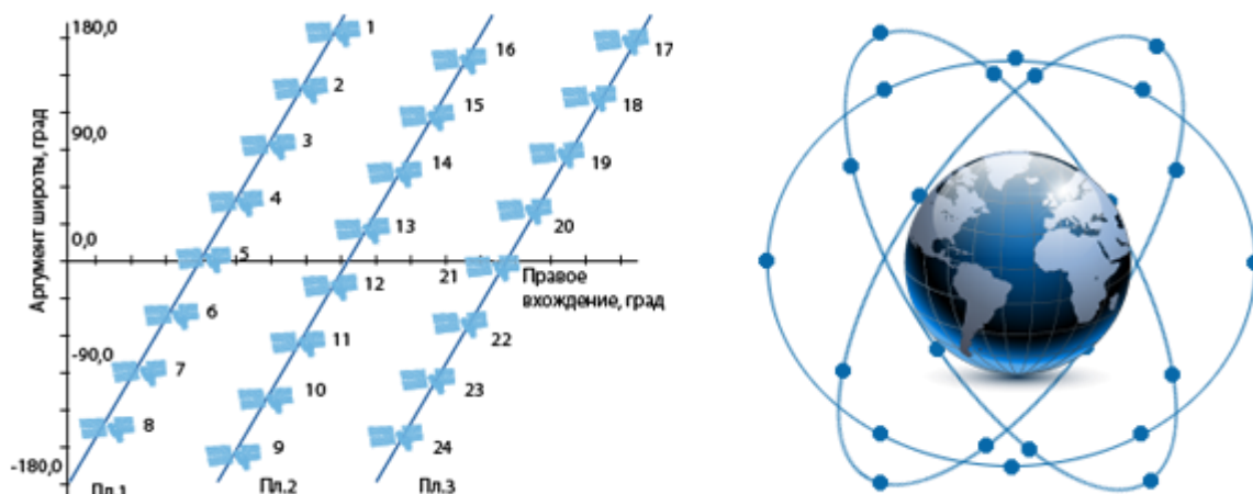
Рисунок 1 – Орбитальное положение спутников на орбитальных плоскостях
