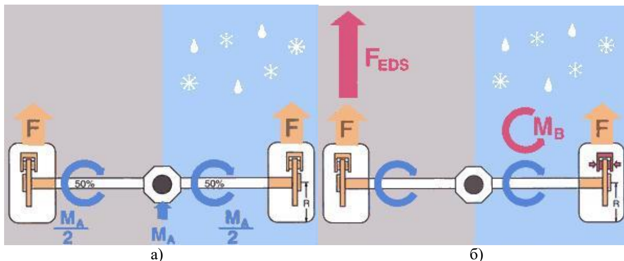
Рисунок 11 – Схема распределения крутящего момента между ведущими колёсами на покрытиях с разным коэффициентом сцепления: а) система не активна; б) система активна – производится при торможении правого колеса.
