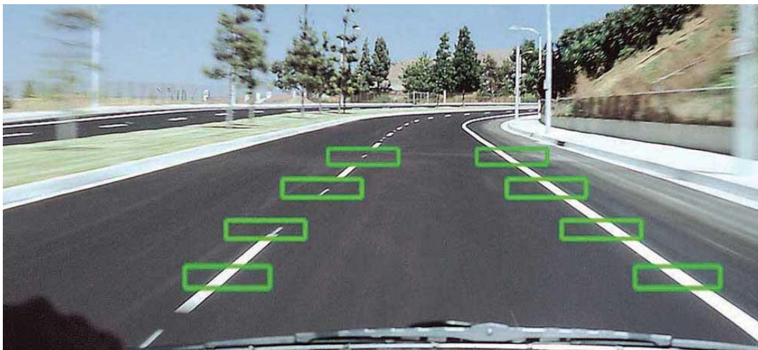
Рисунок 10 – Работа монохромной камеры, в процессе распознавания линии разметки как резкого изменения градации серого.
