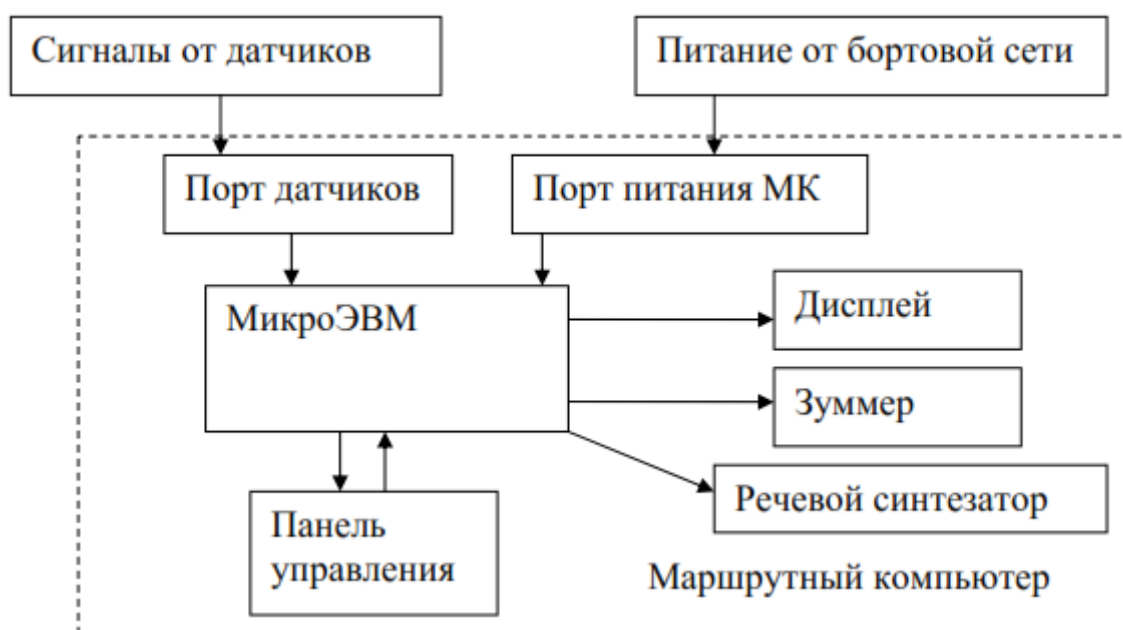
Рисунок 3 - Структурная схема автомобильного маршрутного компьютера
