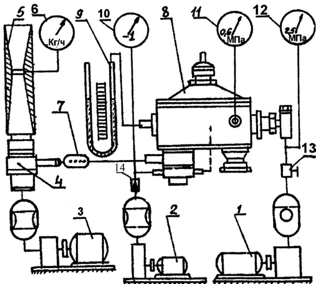
Рис. 5.1. Схема устройства безмоторного стенда: 1- компрессор ГАРО; 2-вакуумный насос высокого давления РВН-20; 3-вакуумный насос низкого давления большой производительности УВН-49; 4- карбюратор-смеситель; 5,6-труба Вентури для измерения расхода воздуха; 7- газовый счетчик (ротаметр РС-5) для измерения расхода газа; 8 - редуктор РЗАА; 9 - пьезометр водяной; 10 - вакуумметр; 11- манометр 0,4 МПа; 12- манометр 2,5 МПа; 13 - вентиль подачи расхода воздуха от компрессора; 14 - вентиль регулировочный.
