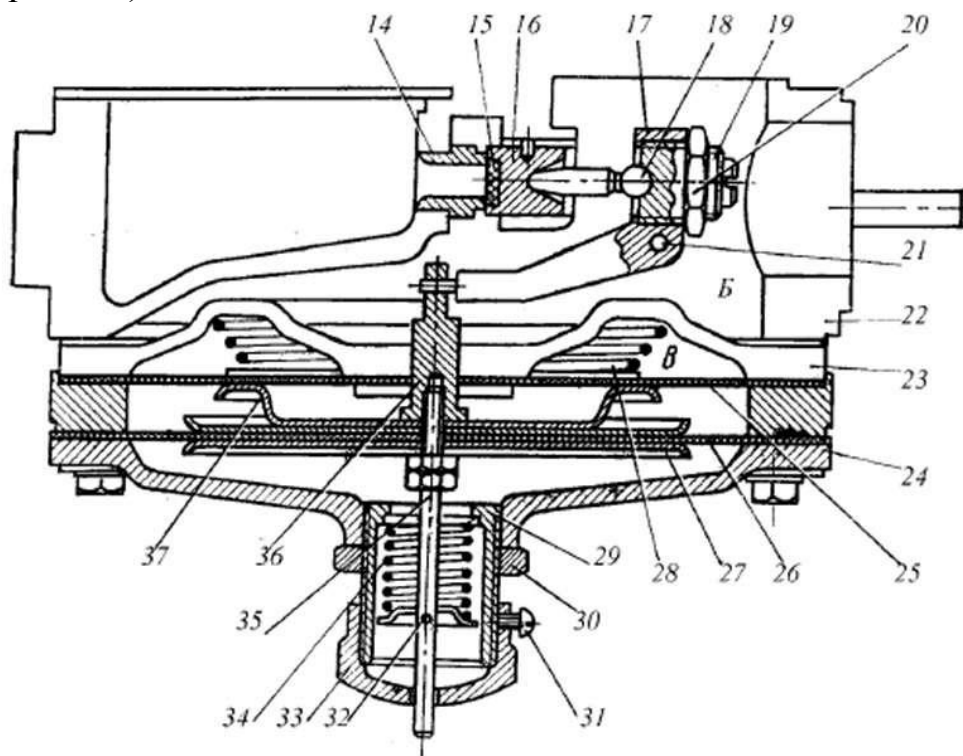
Рис. 3.3. Вторая ступень редуктора РЗД: 14 - седло клапана; 15 - уплотнитель; 16 - клапан низкого давления; 17 - рычаг клапана второй ступени; 18 - толкатель клапана; 19 - регулировочный винт; 20 – контргайка; 21 – ось; 22 - корпус ре-
