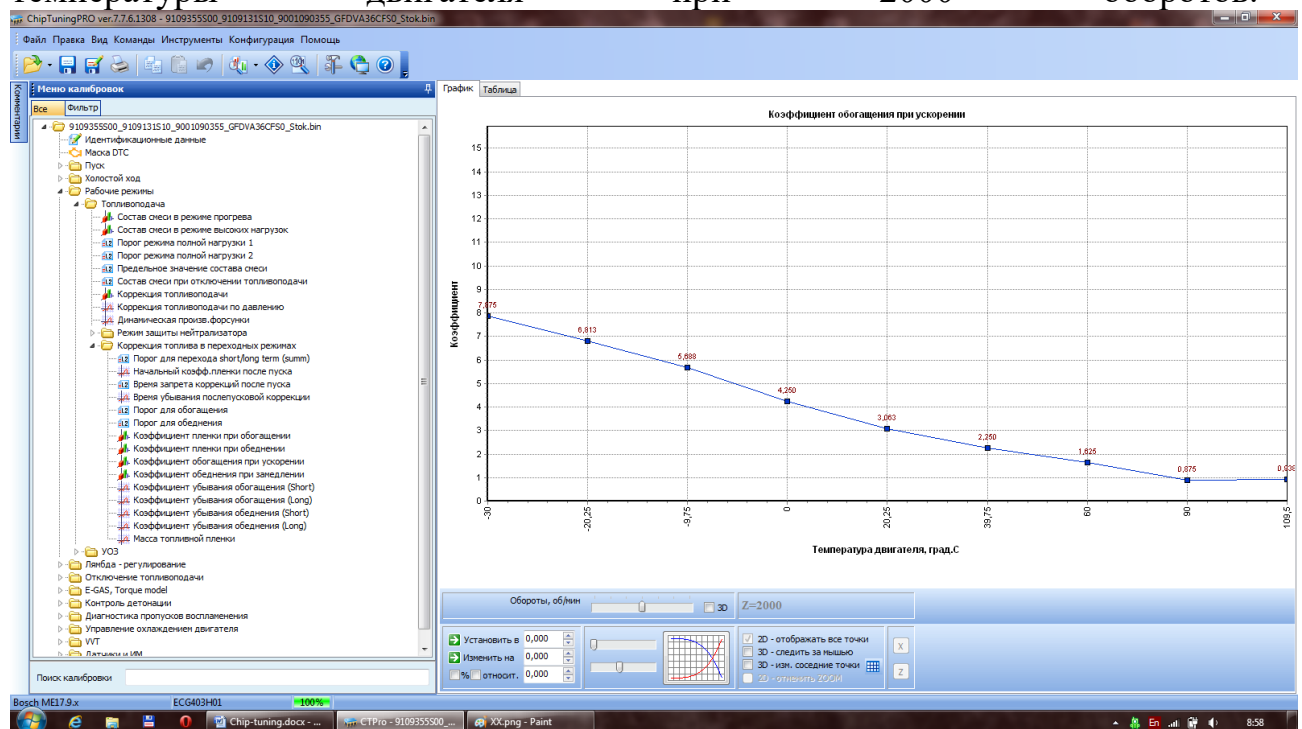
Рисунок 11. Коэффициент обогащения при ускорении в зависимости от температуры двигателя при 2000 оборотах.
