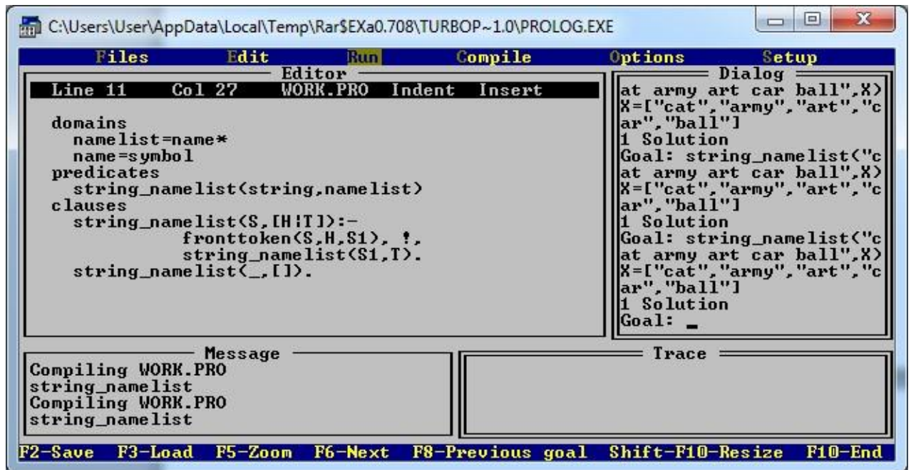
Рисунок 7.2 – Пример программы
