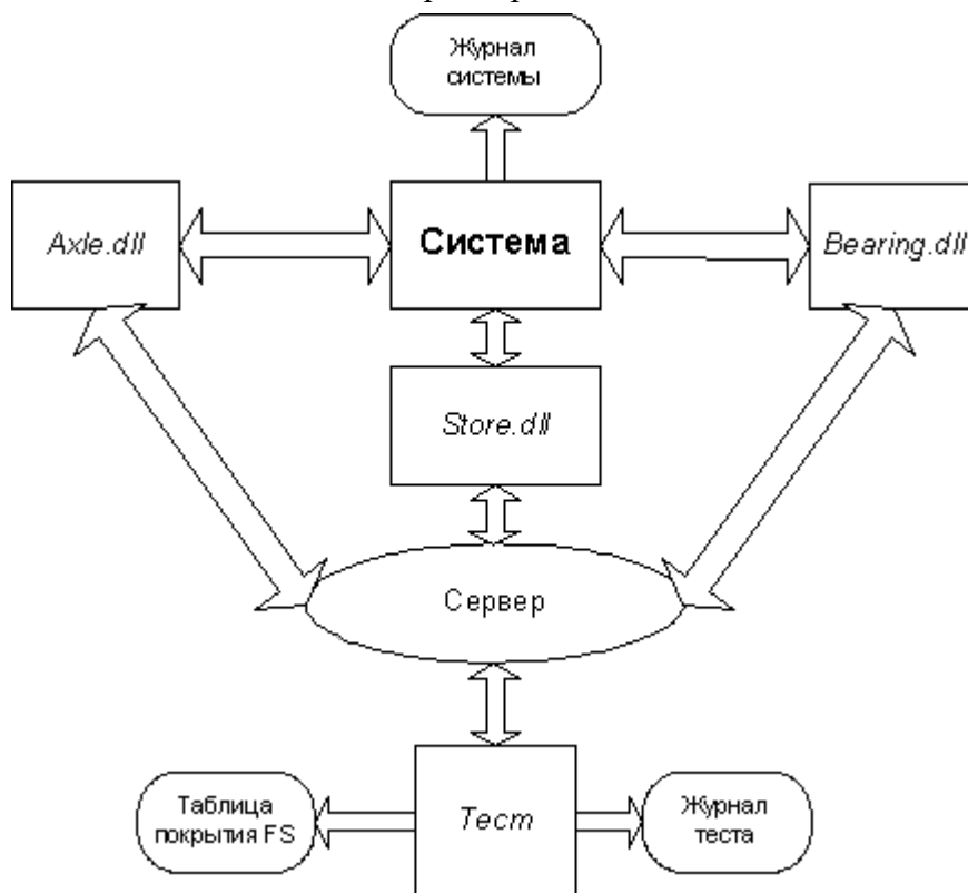
Рис. 6.1. Система и ее окружение (скрипты) source bin\\
