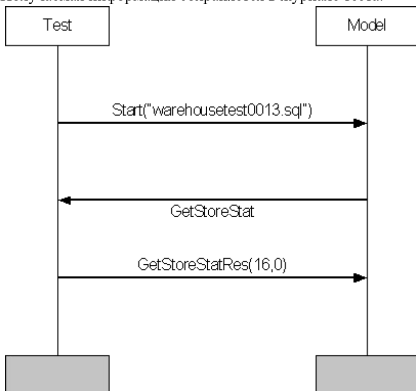
Рис. 7.2. Взаимодействие теста и модели (MSC-диаграмма)
