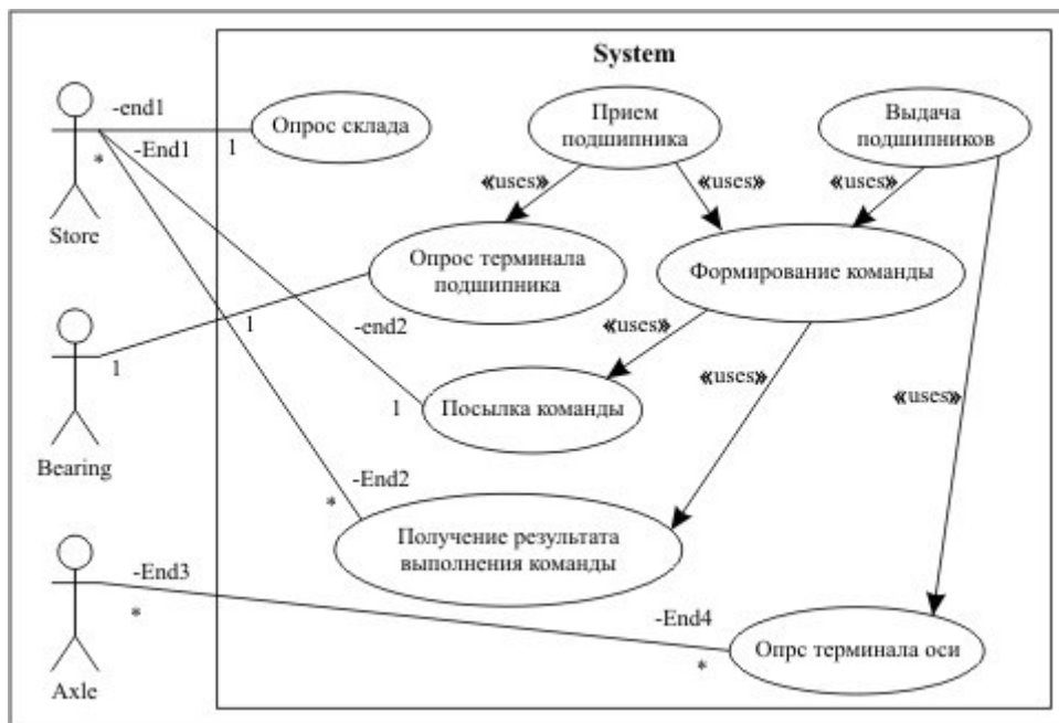
Рис. 14.1. Use case-диаграмма
